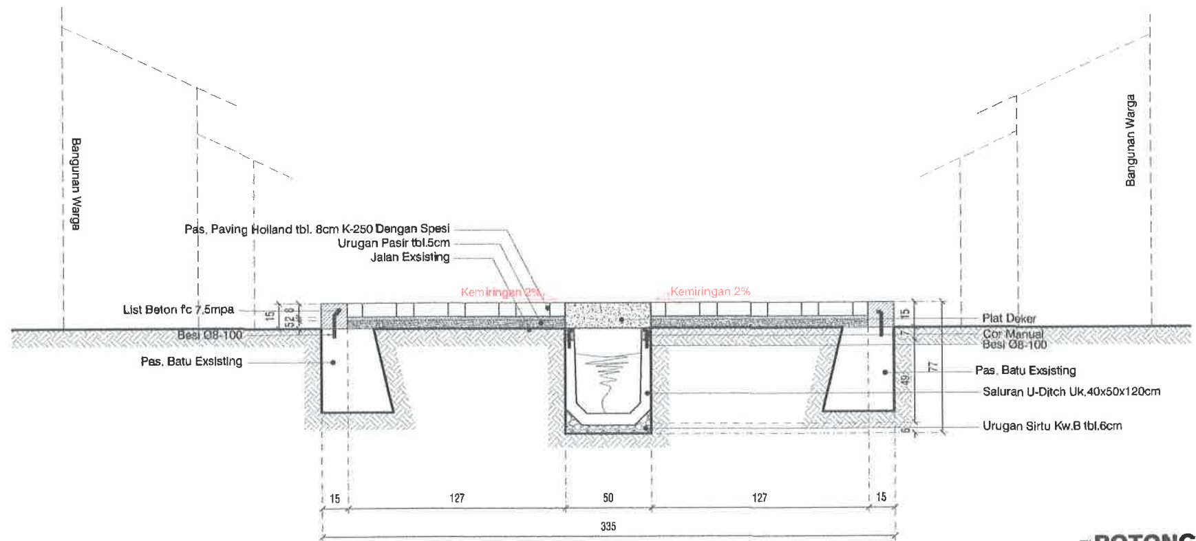
POTONGAN STA 0+275
