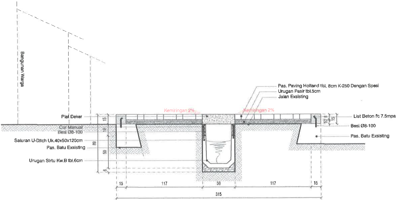
POTONGAN STA 0+075 SKALA 1 : 30
