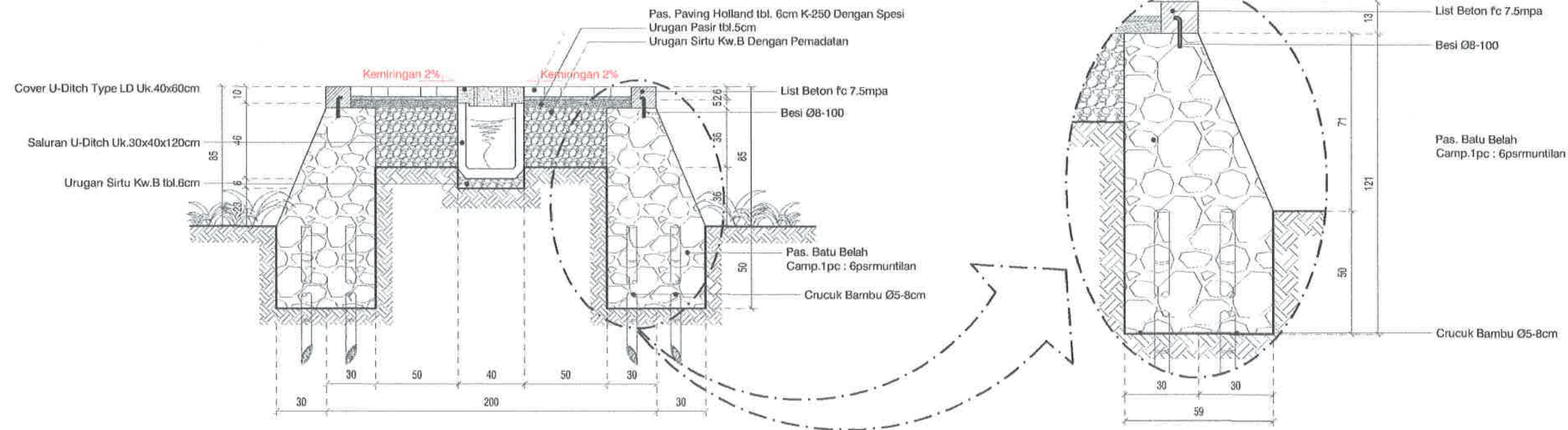
POTONGAN STA 0+000 SKALA 1 : 30
