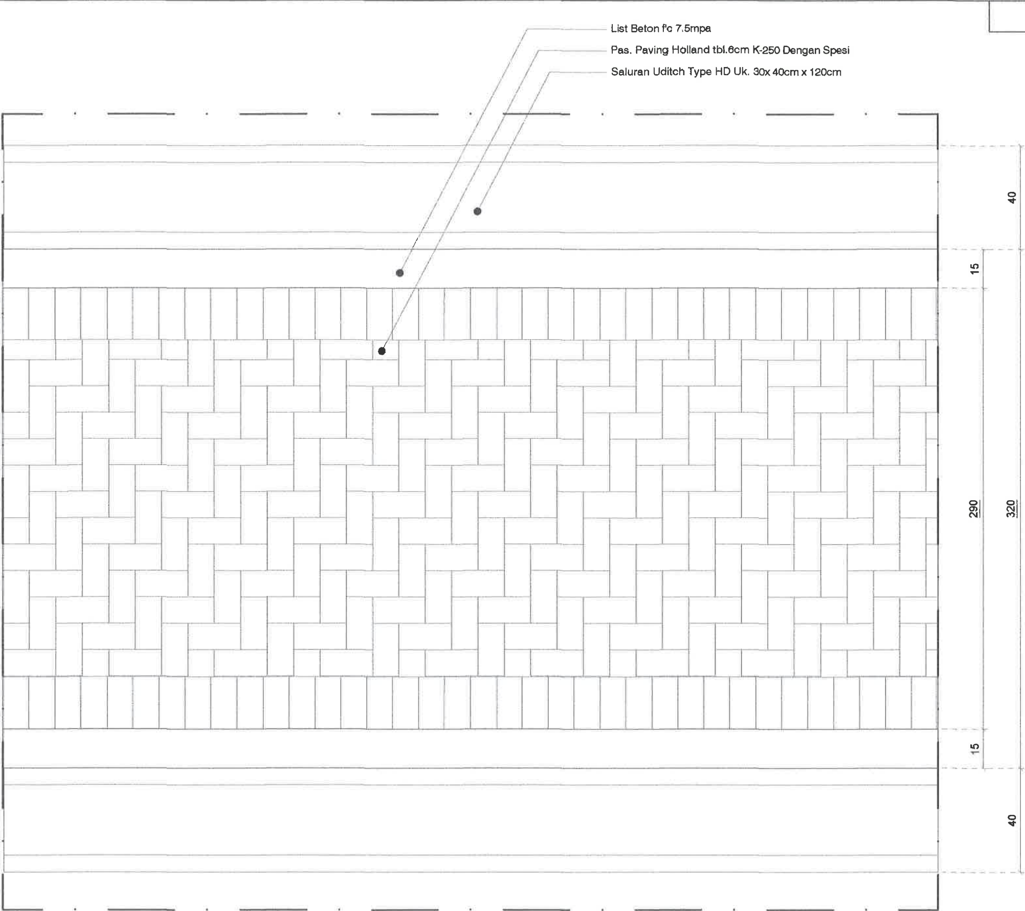
DETAIL MOTIF PAVING SKALA 1 : 15
