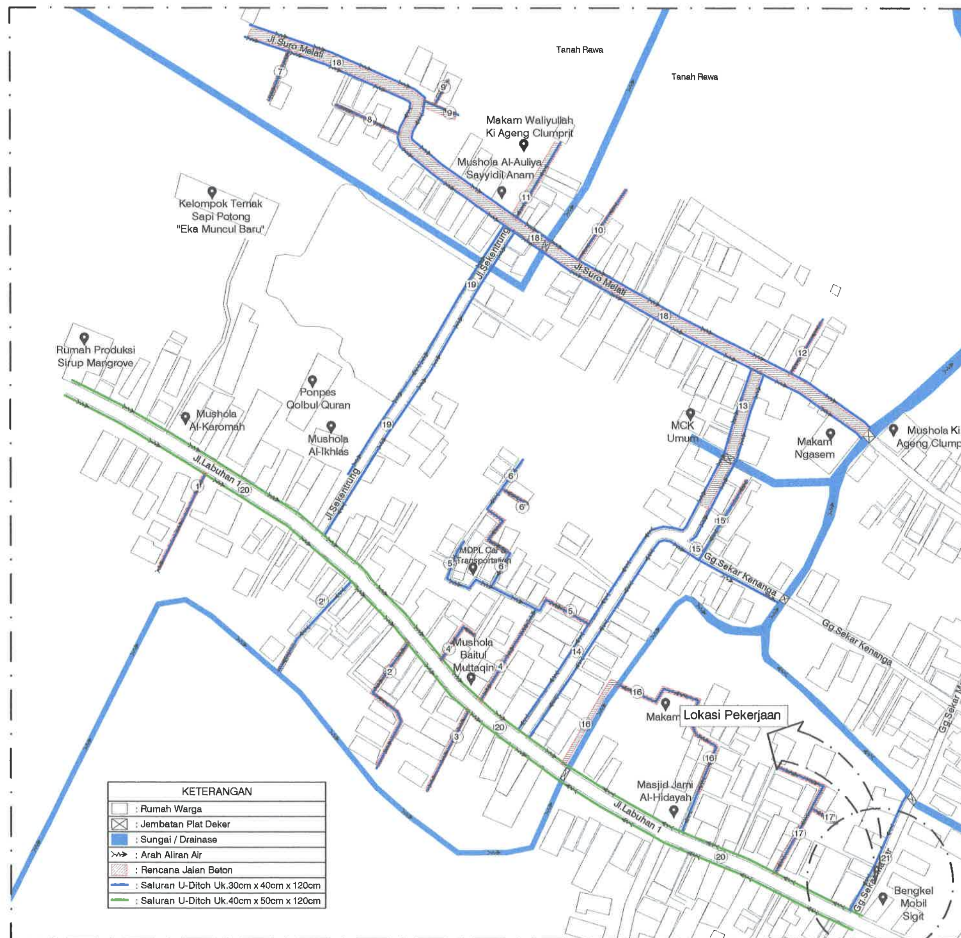
SITEPLAN RENCANA SALURAN DRAINASE 21 SKALA : Nts
