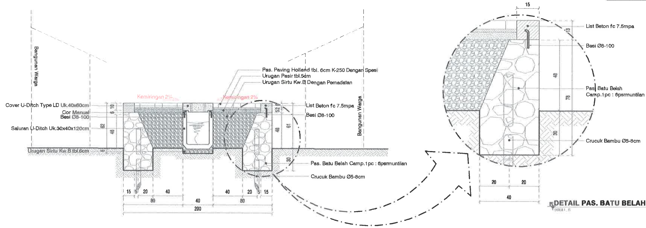
POTONGAN STA 0+020 SKALA 1 : 30
