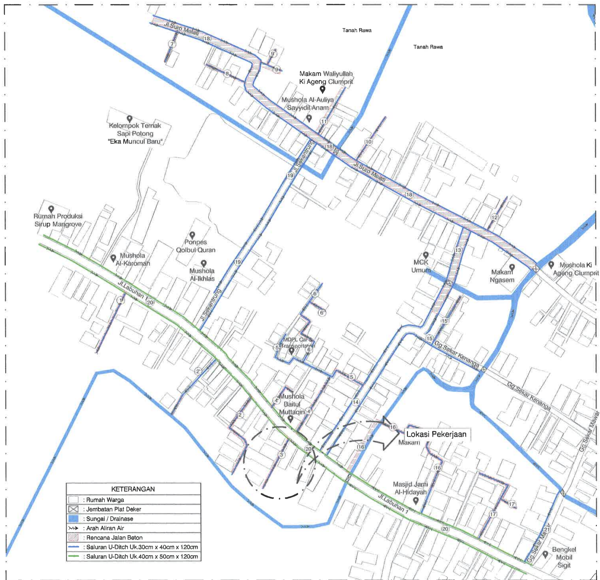
SITEPLAN RENCANA JALAN SALURAN DRAINASE RUAS 3 SKALA : Nis
