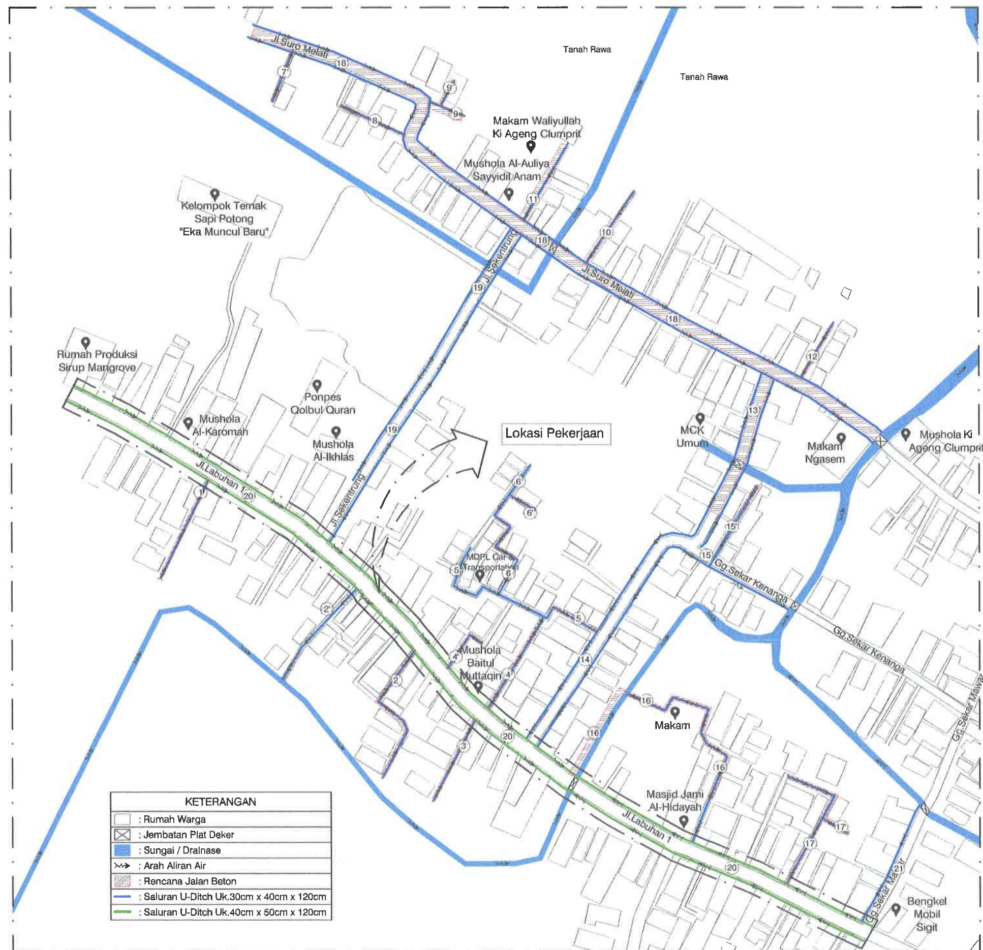
SITEPLAN RENCANA SALURAN DRAINASE RUAS 20 SKALA : Nts
