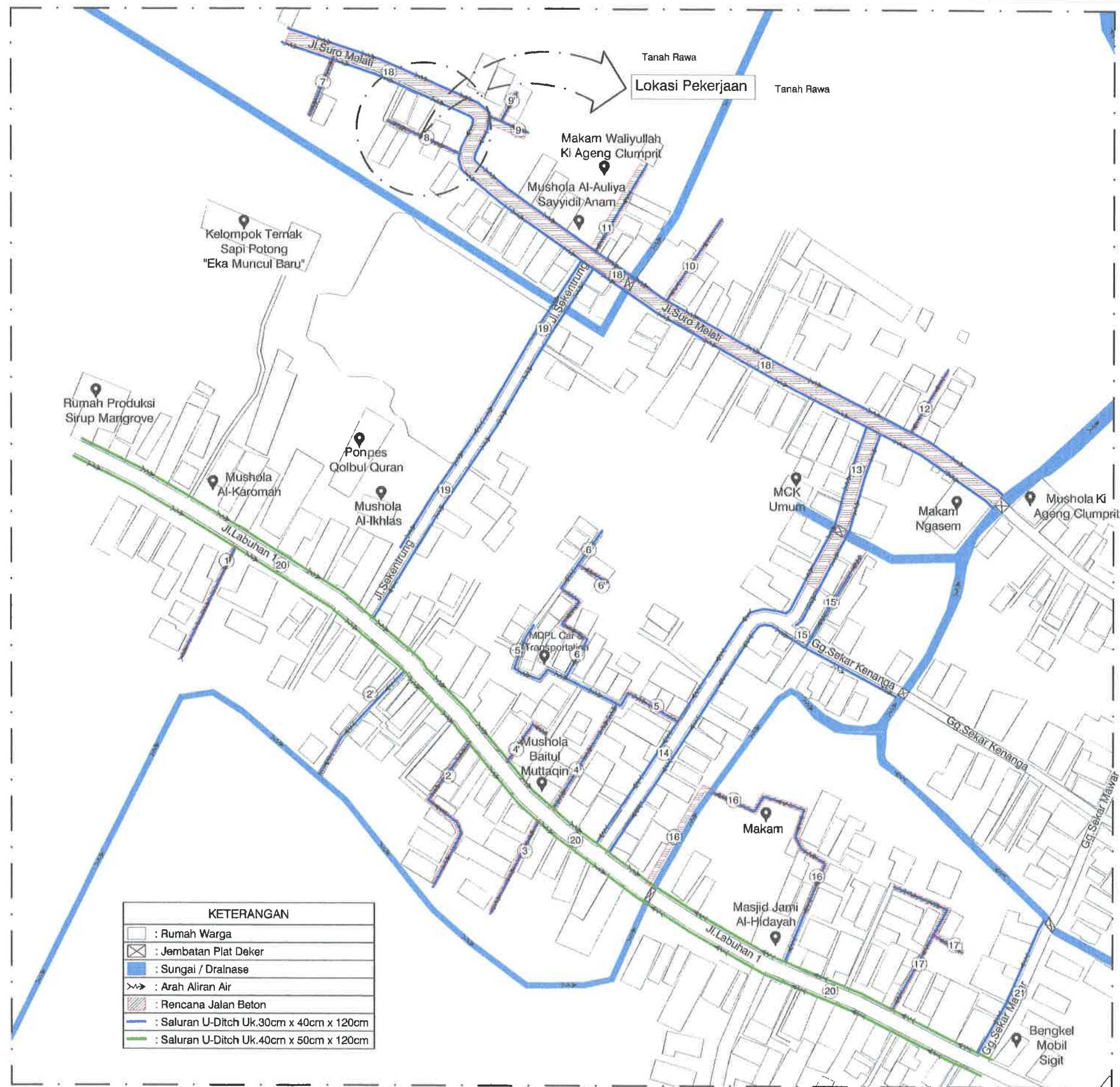
SITEPLAN RENCANA JALAN SALURAN DRAINASE RUAS 8 SKALA : Nis
