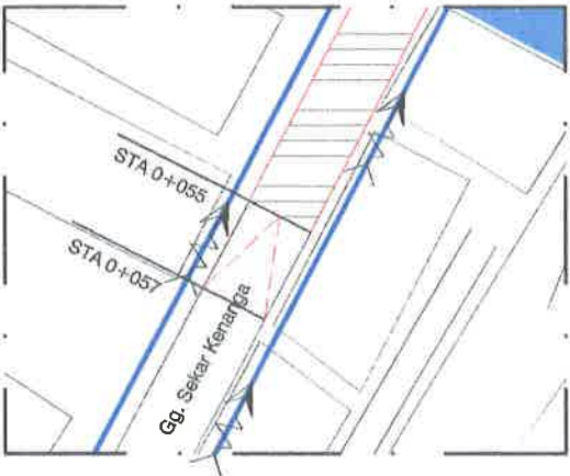
DENAH OPRITAN AKHIR SKALA : Nis
