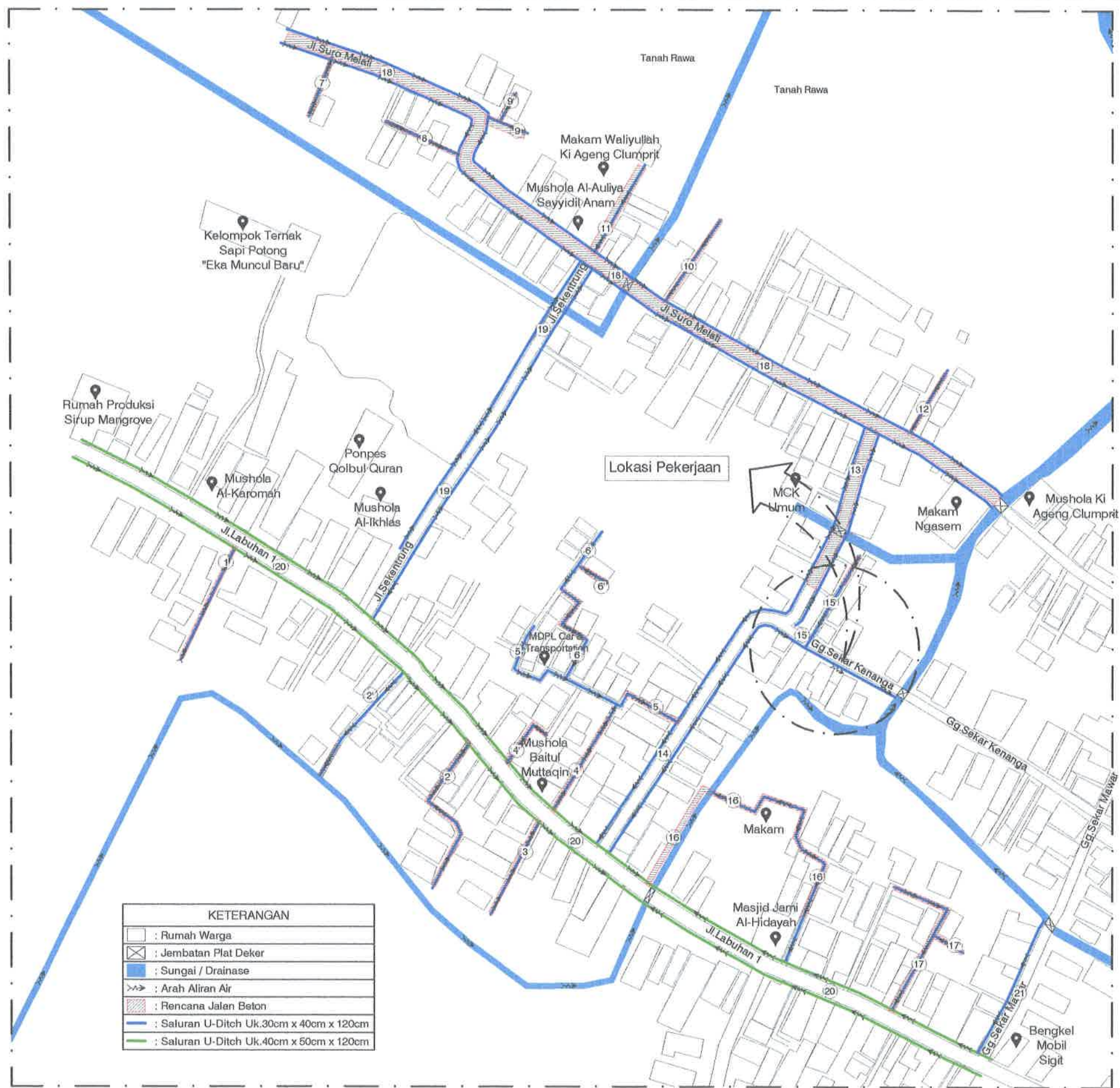
SITEPLAN RENCANA JALAN SALURAN DRAINASE RUAS 15 SKALA : Nts
