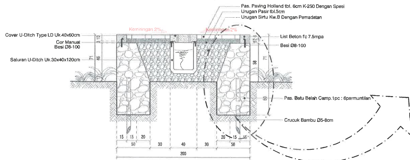
POTONGAN STA 0+039.2
