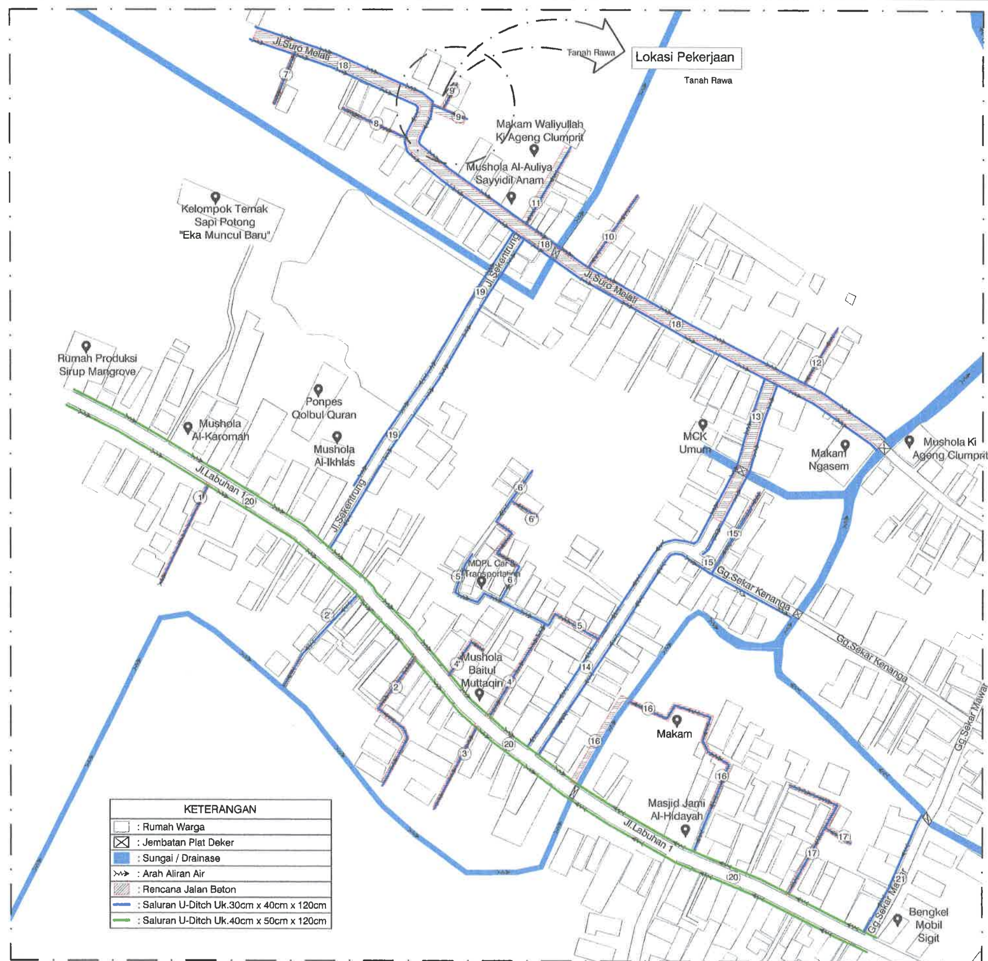
SITEPLAN RENCANA JALAN SALURAN DRAINASE RUAS 9' SKALA : Nts
