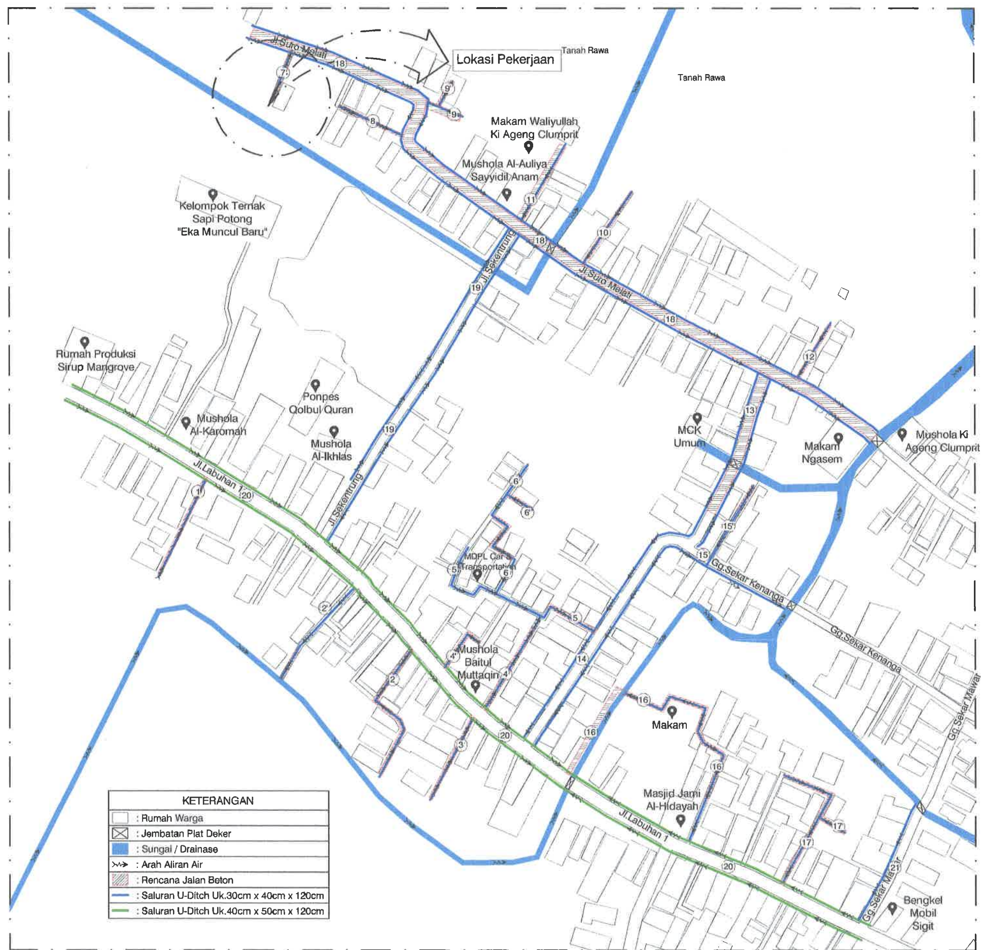
SITEPLAN RENCANA JALAN SALURAN DRAINASE RUAS 7 SKALA : Nis
