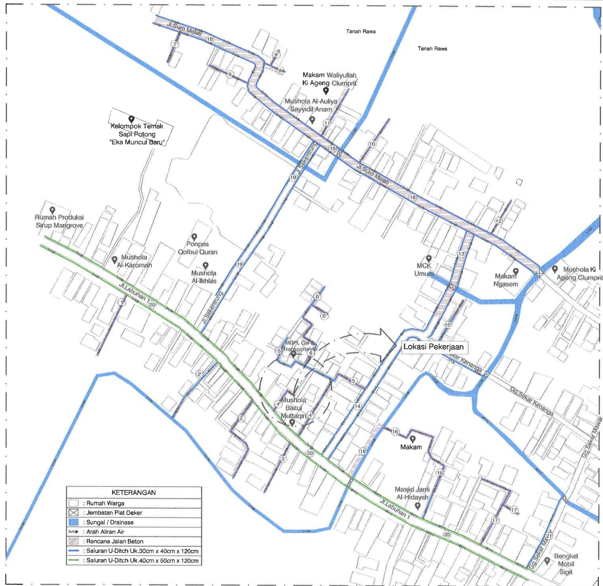
SITEPLAN RENCANA JALAN SALURAN DRAINASE RUAS 4' SKALA : Nis
