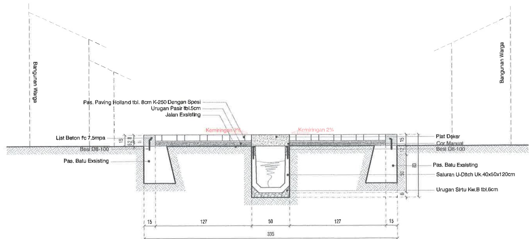
POTONGAN STA 0+300
