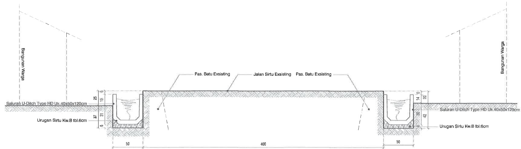
POTONGAN STA 0+300
