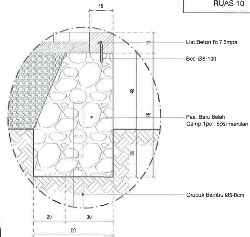
POTONGAN STA 0+016.5
