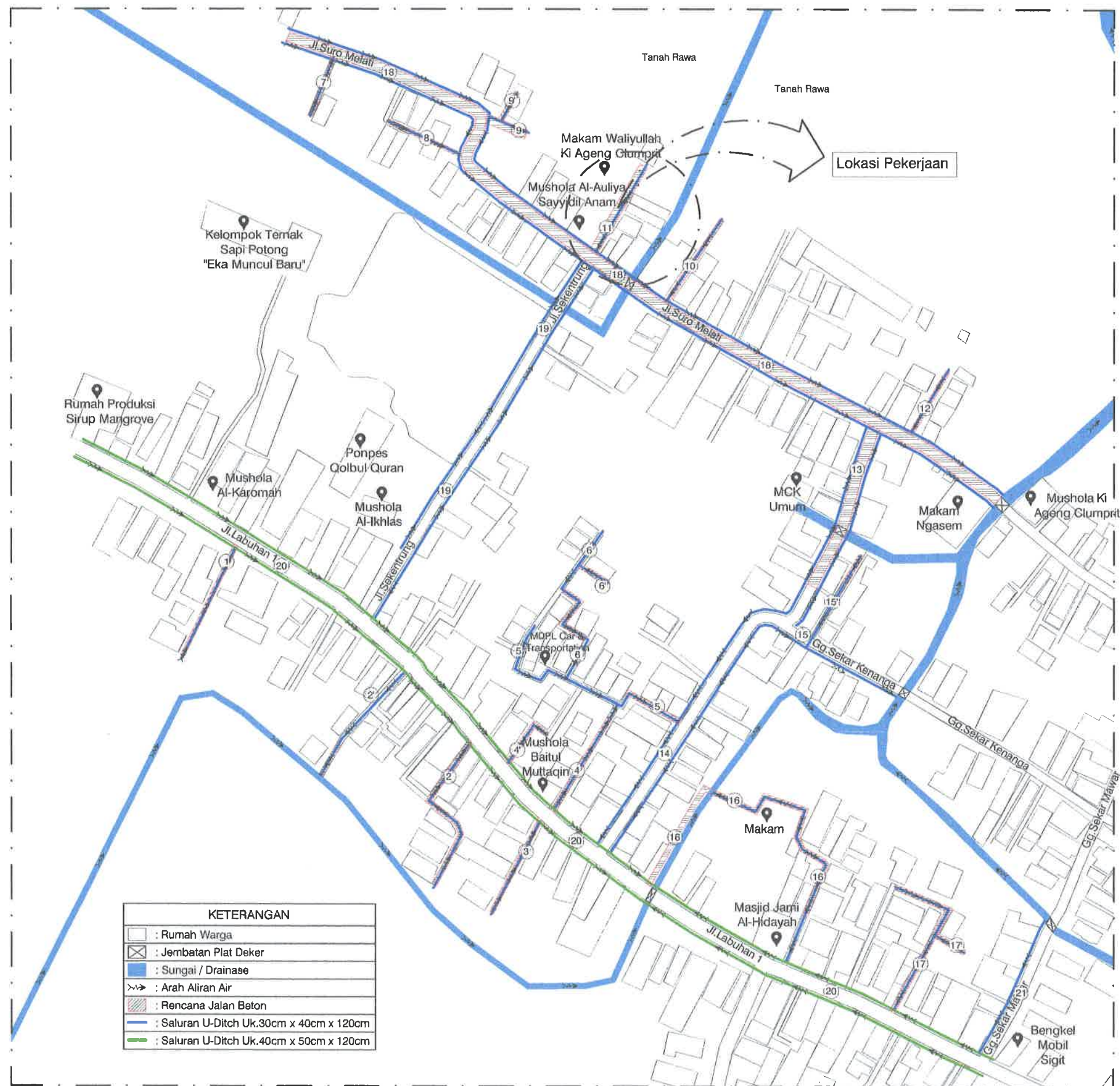
SITEPLAN RENCANA JALAN SALURAN DRAINASE RUAS 11 SKALA : Nis
