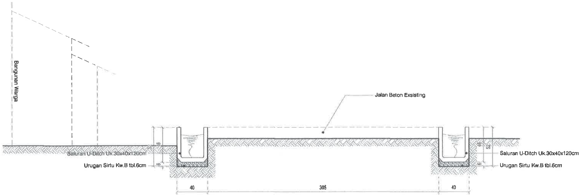
POTONGAN STA 0+000 SKALA 1 : 30
