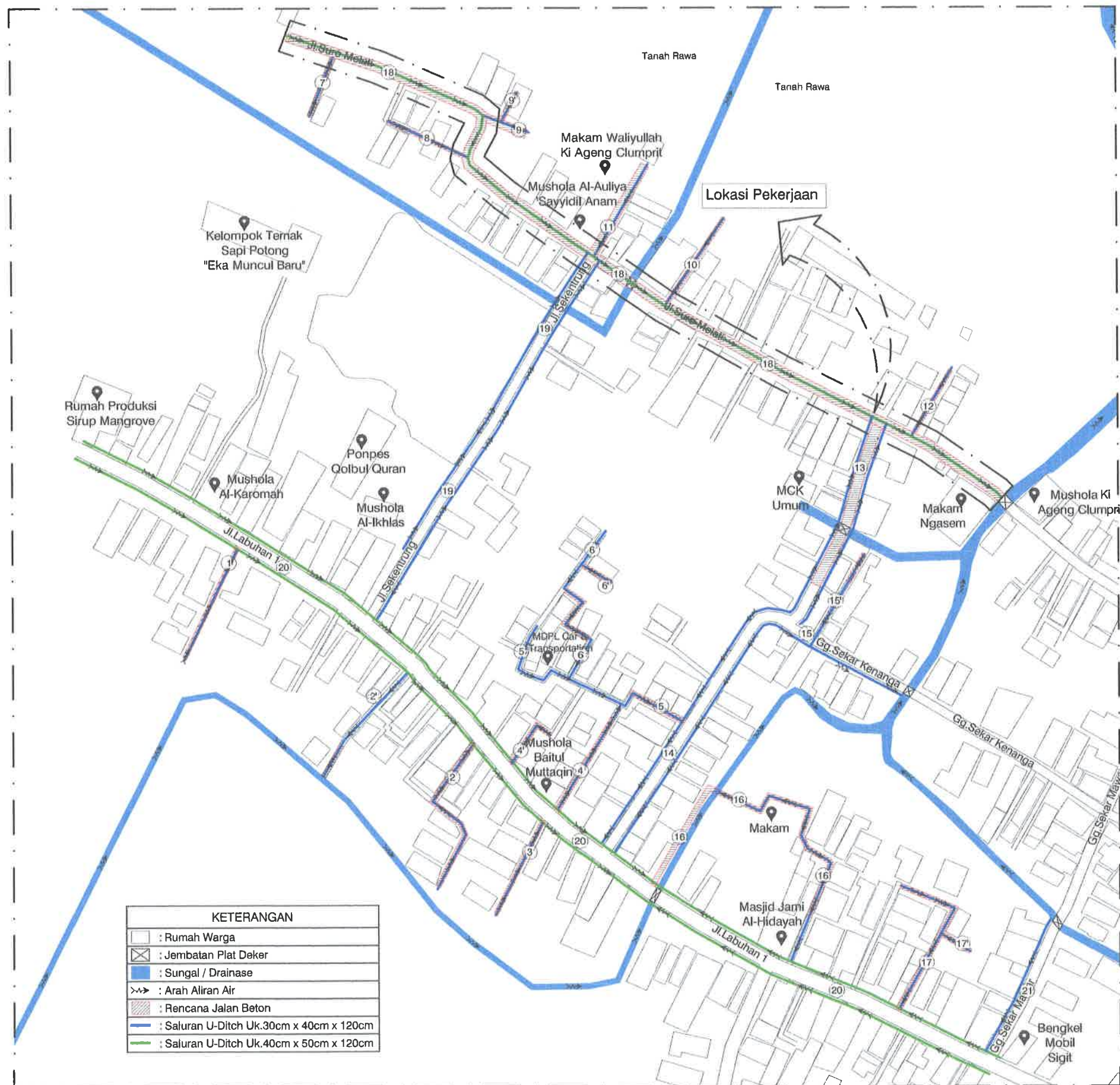
SITEPLAN RENCANA JALAN SALURAN DRAINASE RUAS 18 SKALA : Nis
