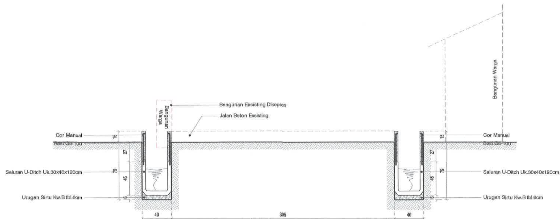
POTONGAN STA 0+000
