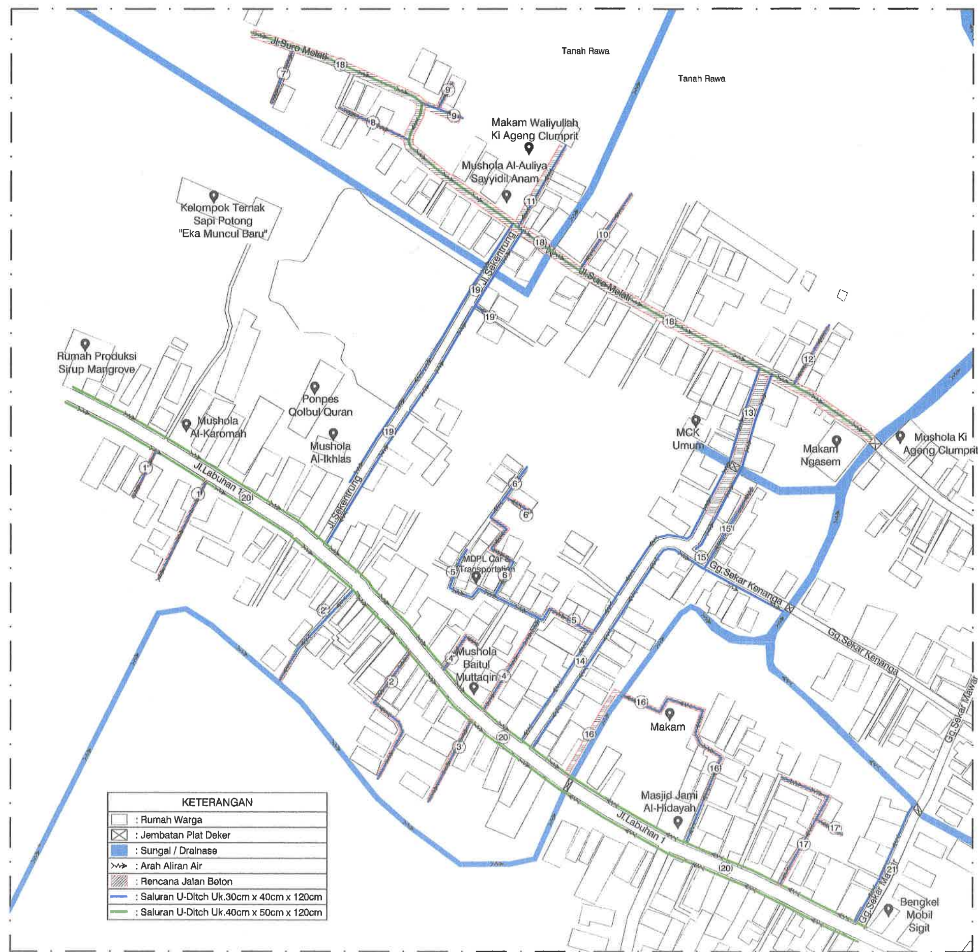
SITEPLAN RENCANA JALAN DAN SALURAN DRAINASE SKALA : Nis
