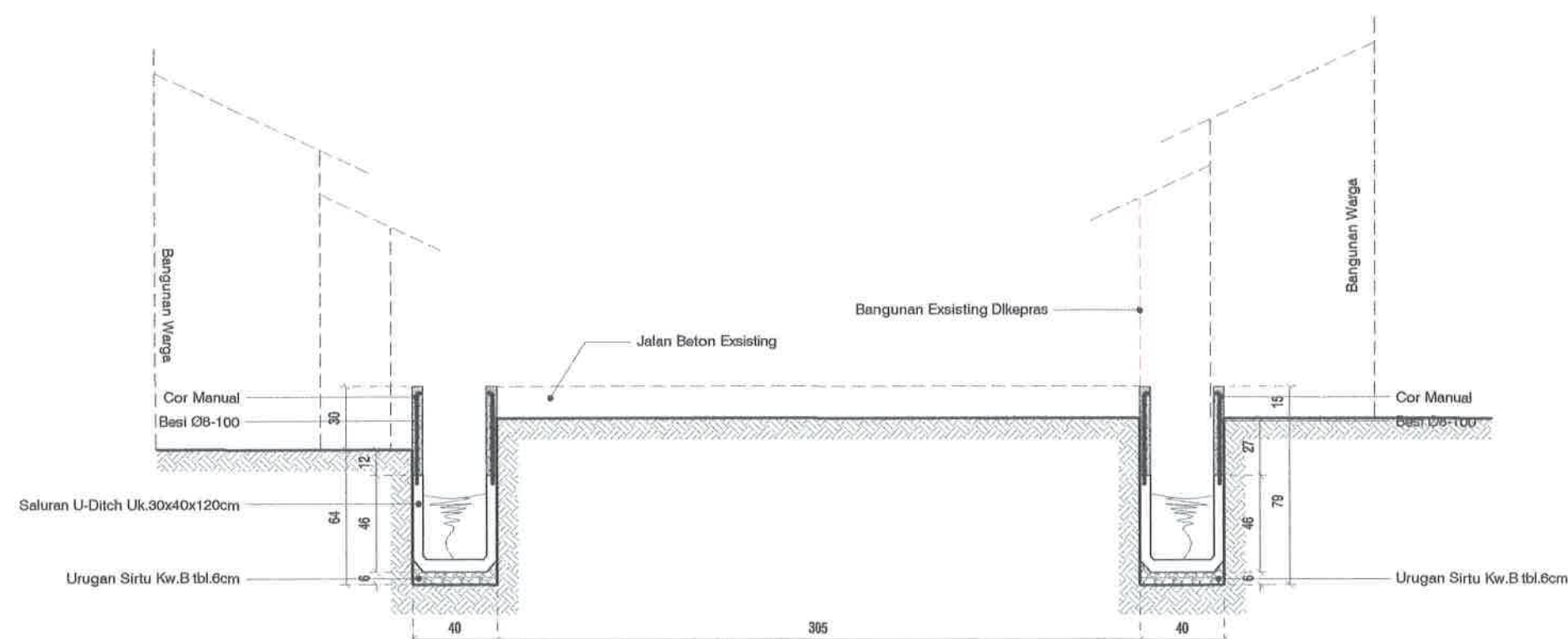
POTONGAN STA 0+008
