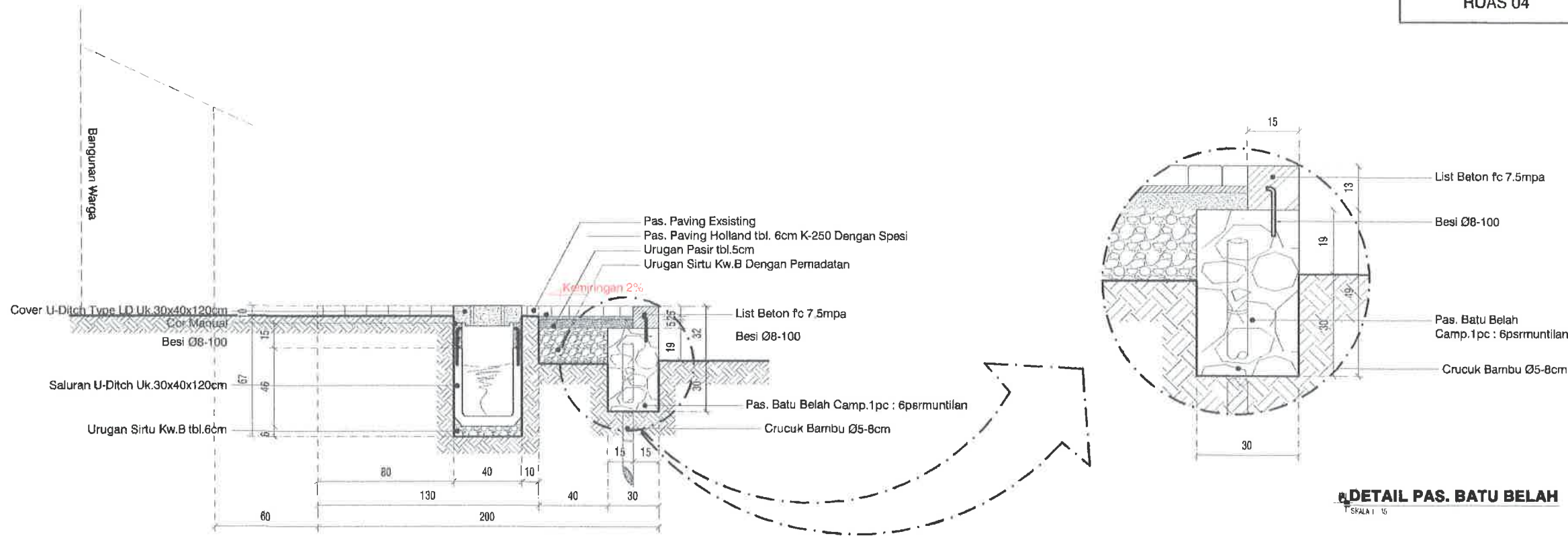
POTONGAN STA 0+005
