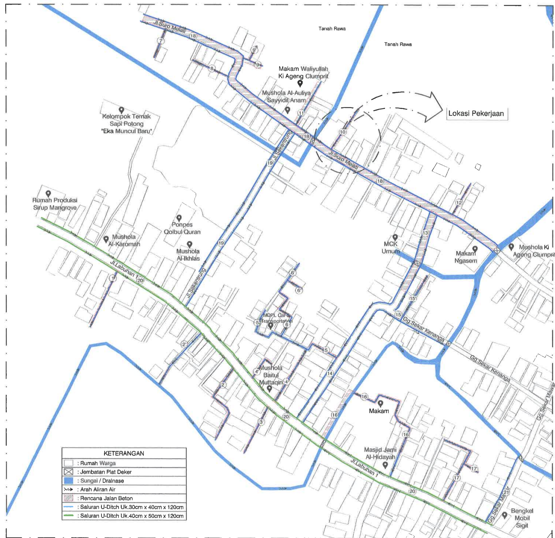
SITEPLAN RENCANA JALAN SALURAN DRAINASE RUAS 10 SKALA : Nts
