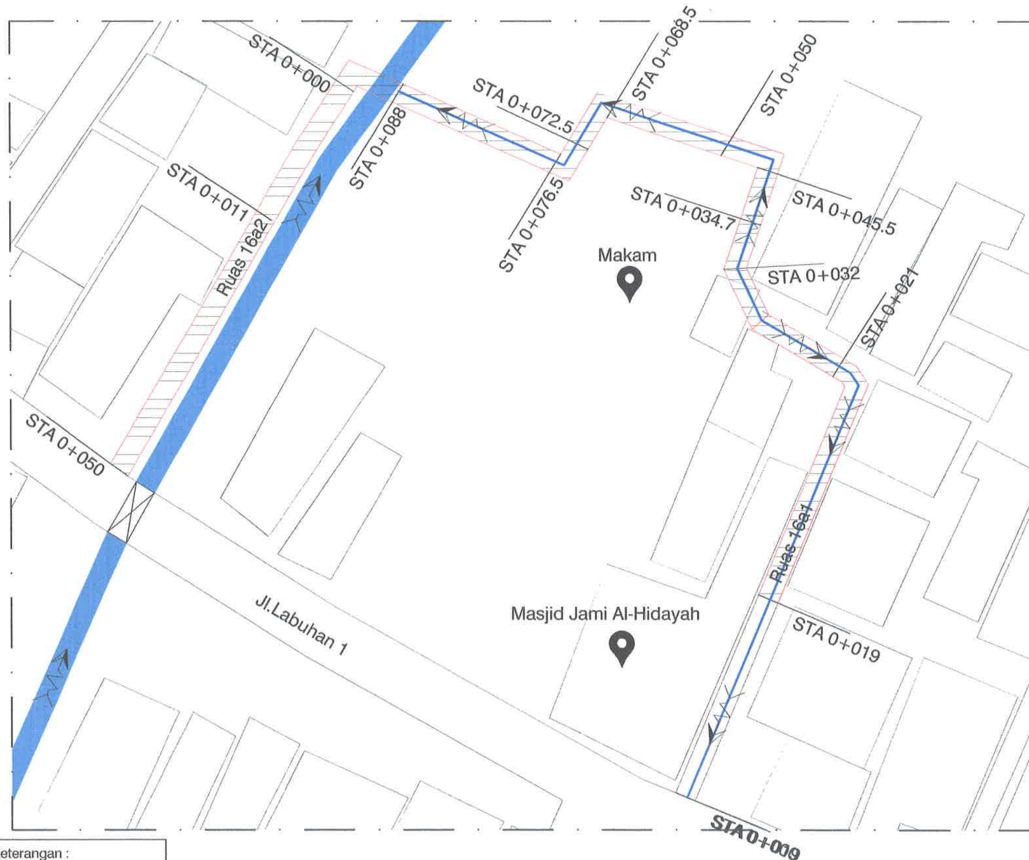
DENAH RENCANA RUAS 16 SKALA : Nis
