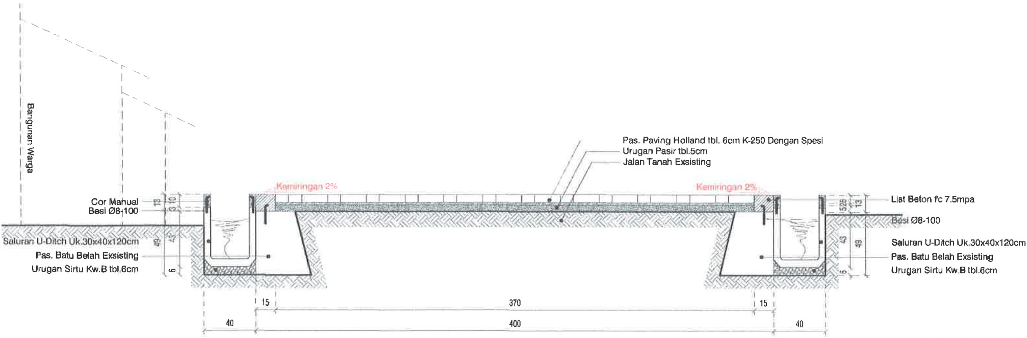
POTONGAN STA 0+000
