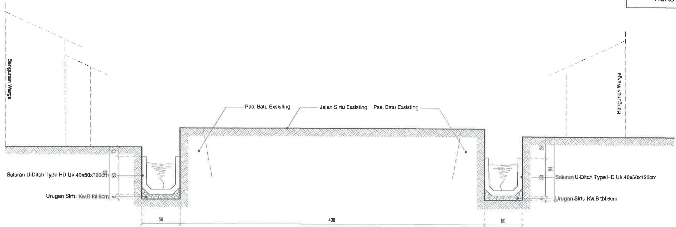
POTONGAN STA 0+100
