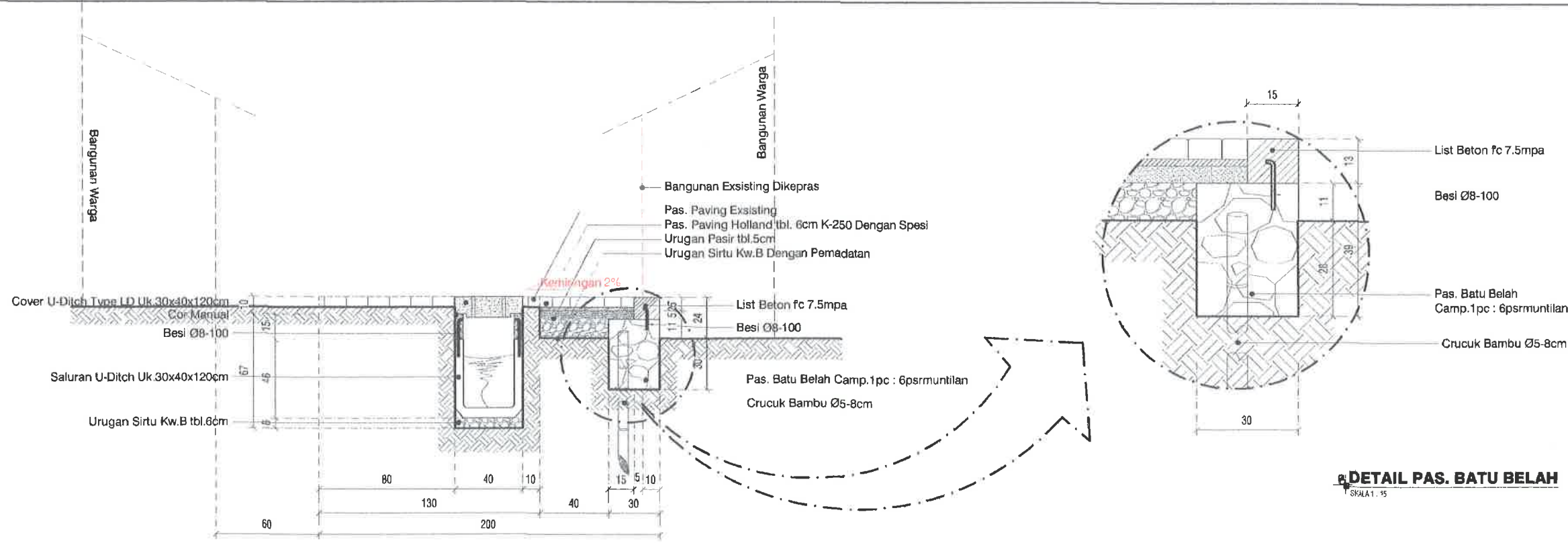
POTONGAN STA 0+005
