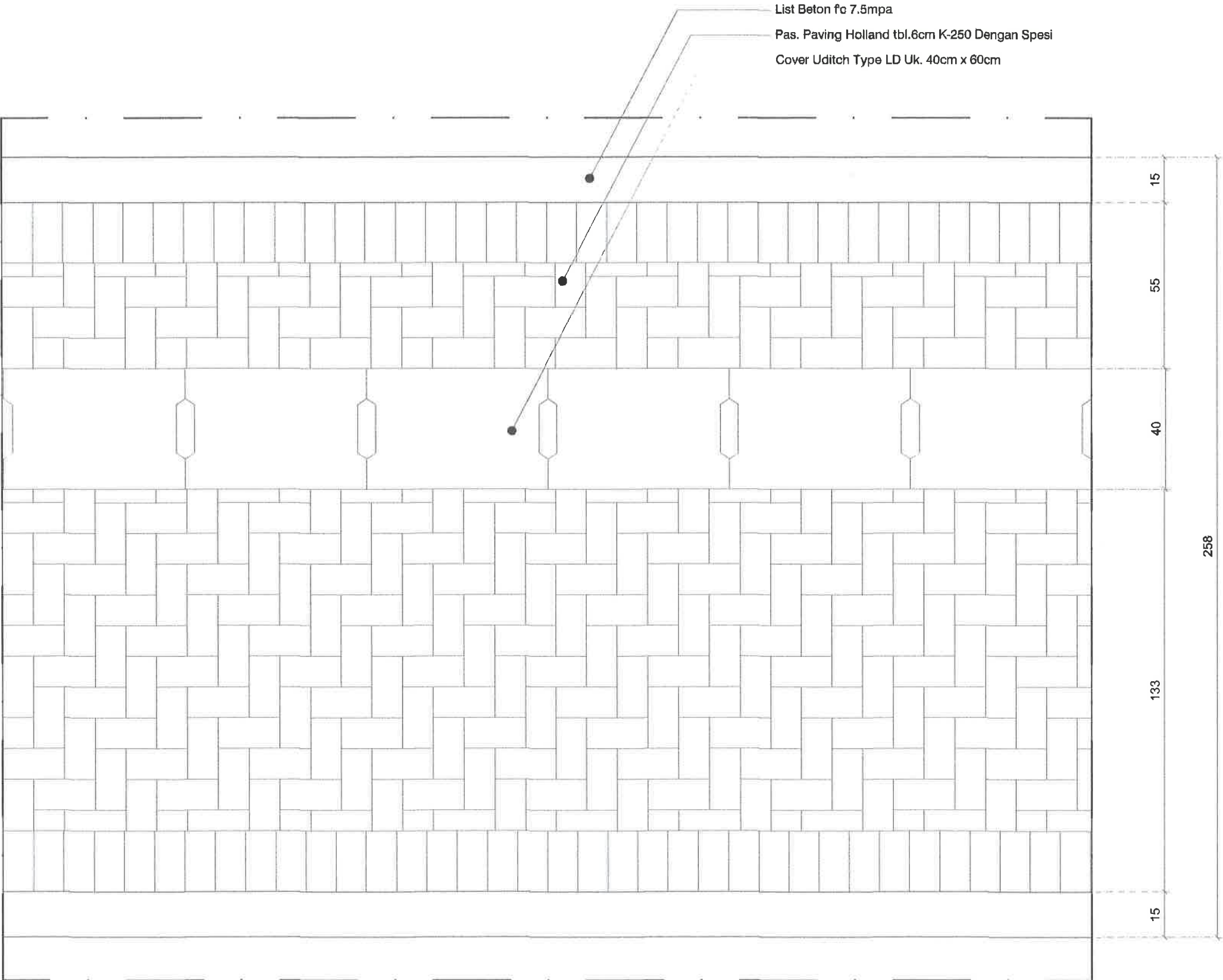
DETAIL MOTIF PAVING SKALA 1 : 15
