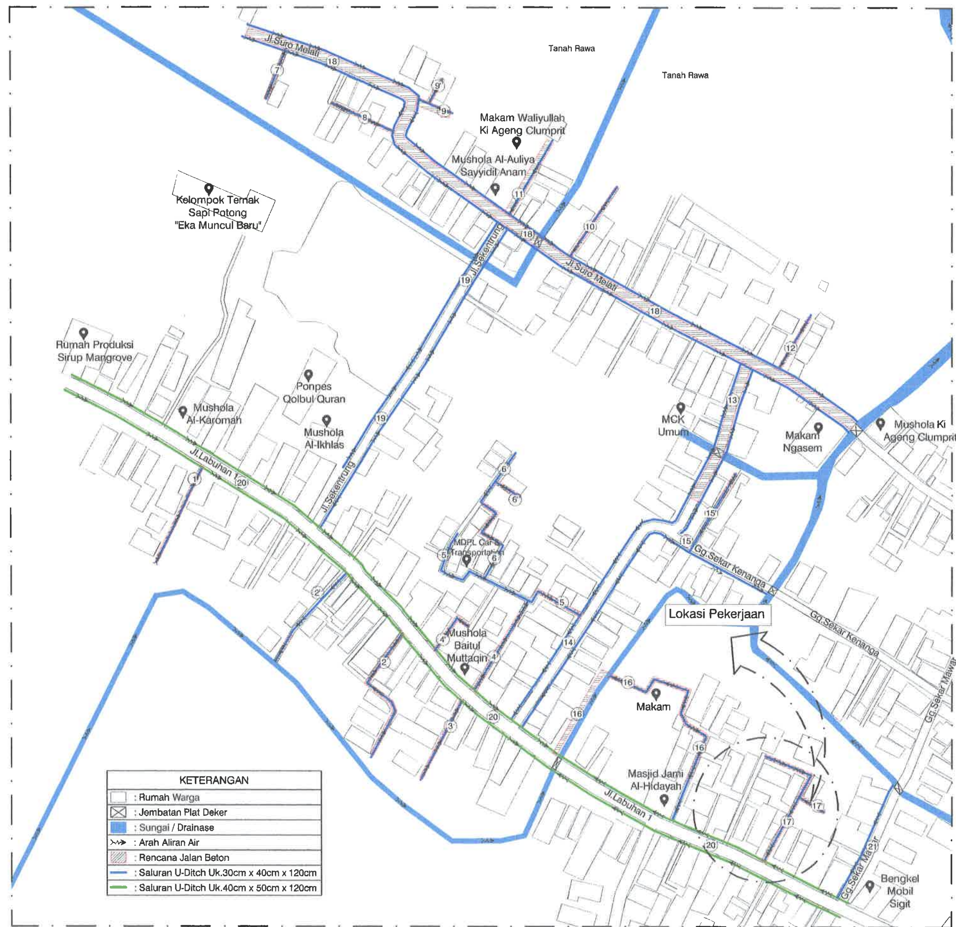
SITEPLAN RENCANA JALAN SALURAN DRAINASE RUAS 17' SKALA : Nts
