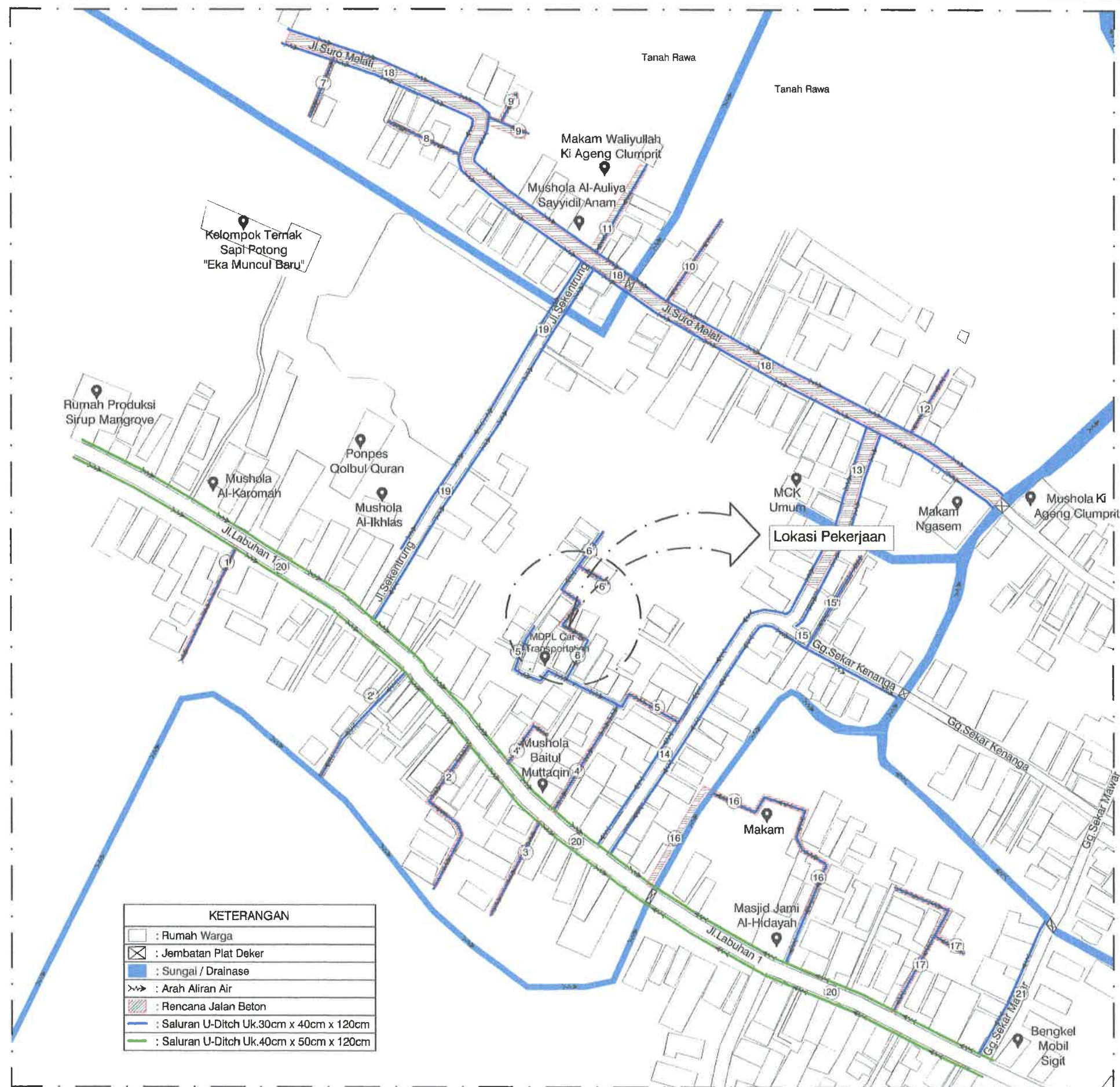
SITEPLAN RENCANA JALAN SALURAN DRAINASE RUAS 6 SKALA : Nis
