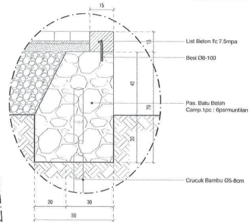
POTONGAN STA 0+000
