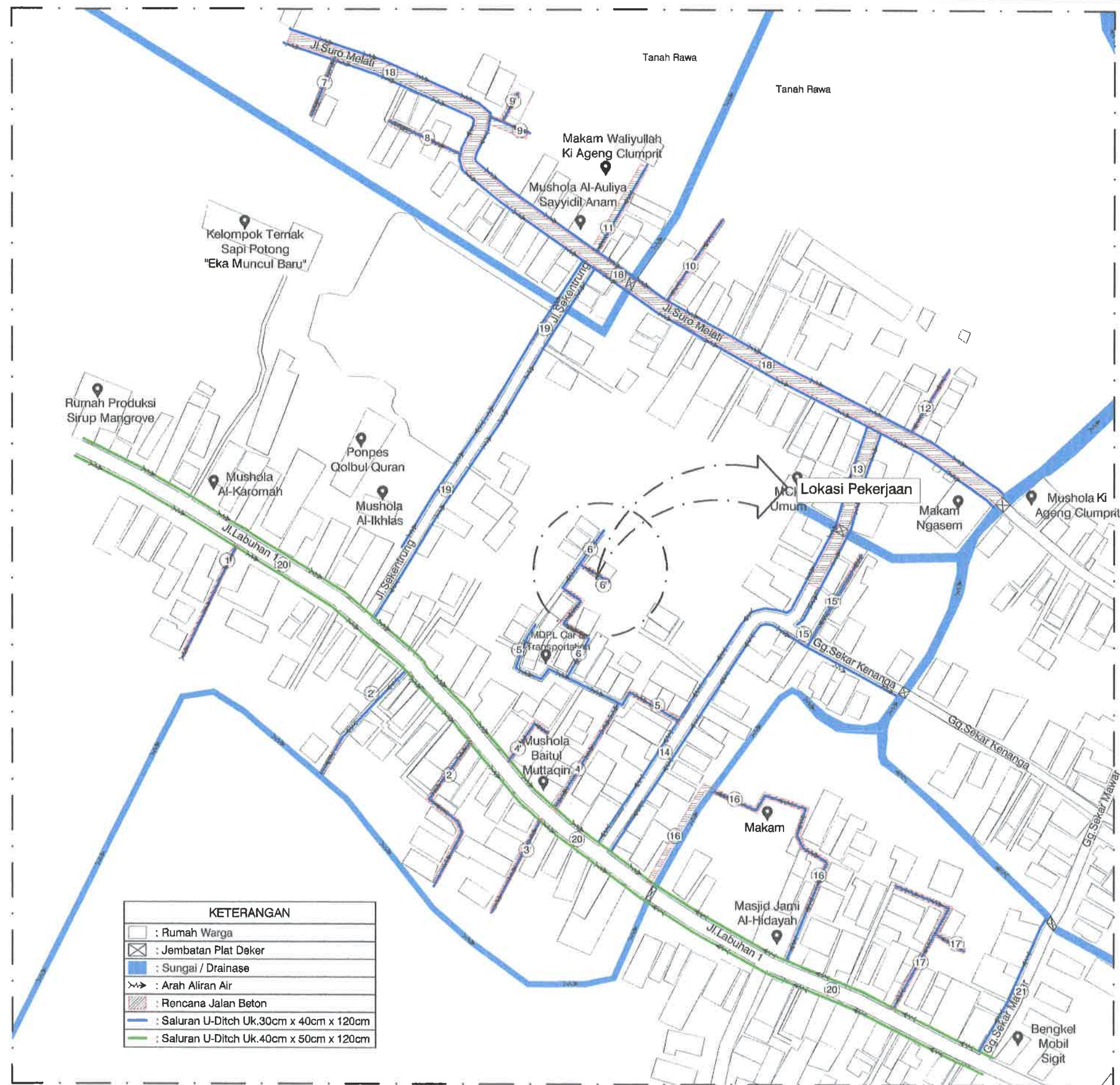
SITEPLAN RENCANA JALAN SALURAN DRAINASE RUAS 6' SKALA : Nts
