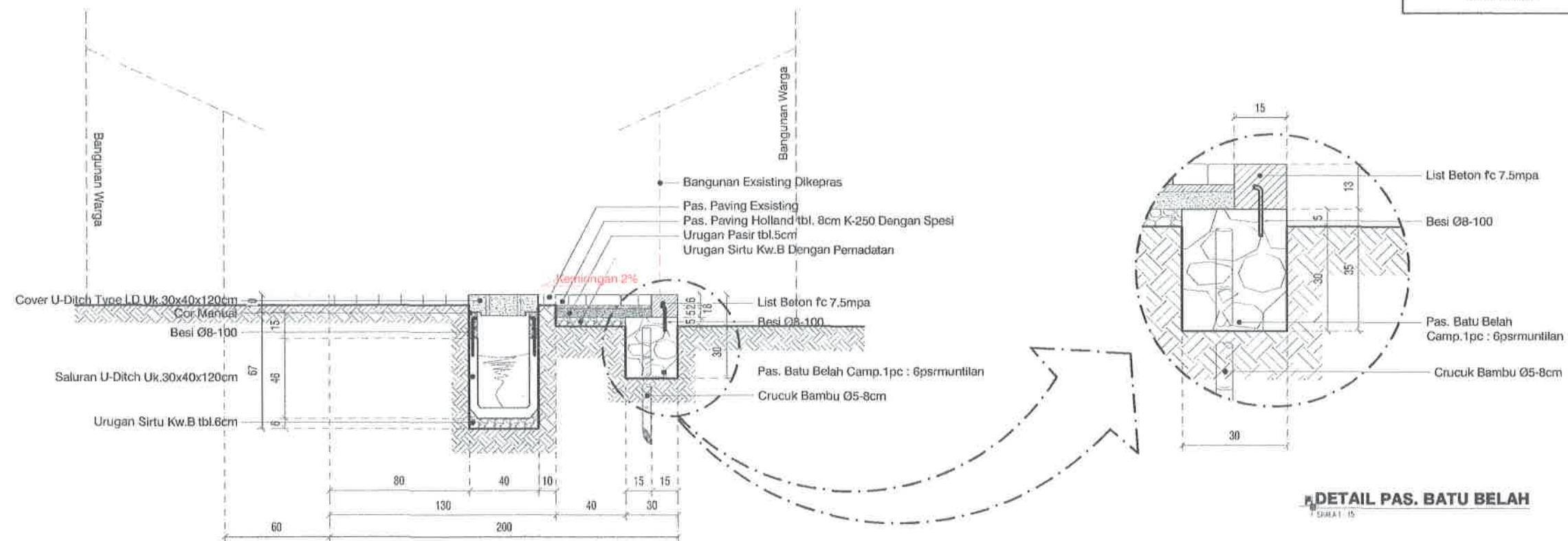
POTONGAN STA 0+028.2
