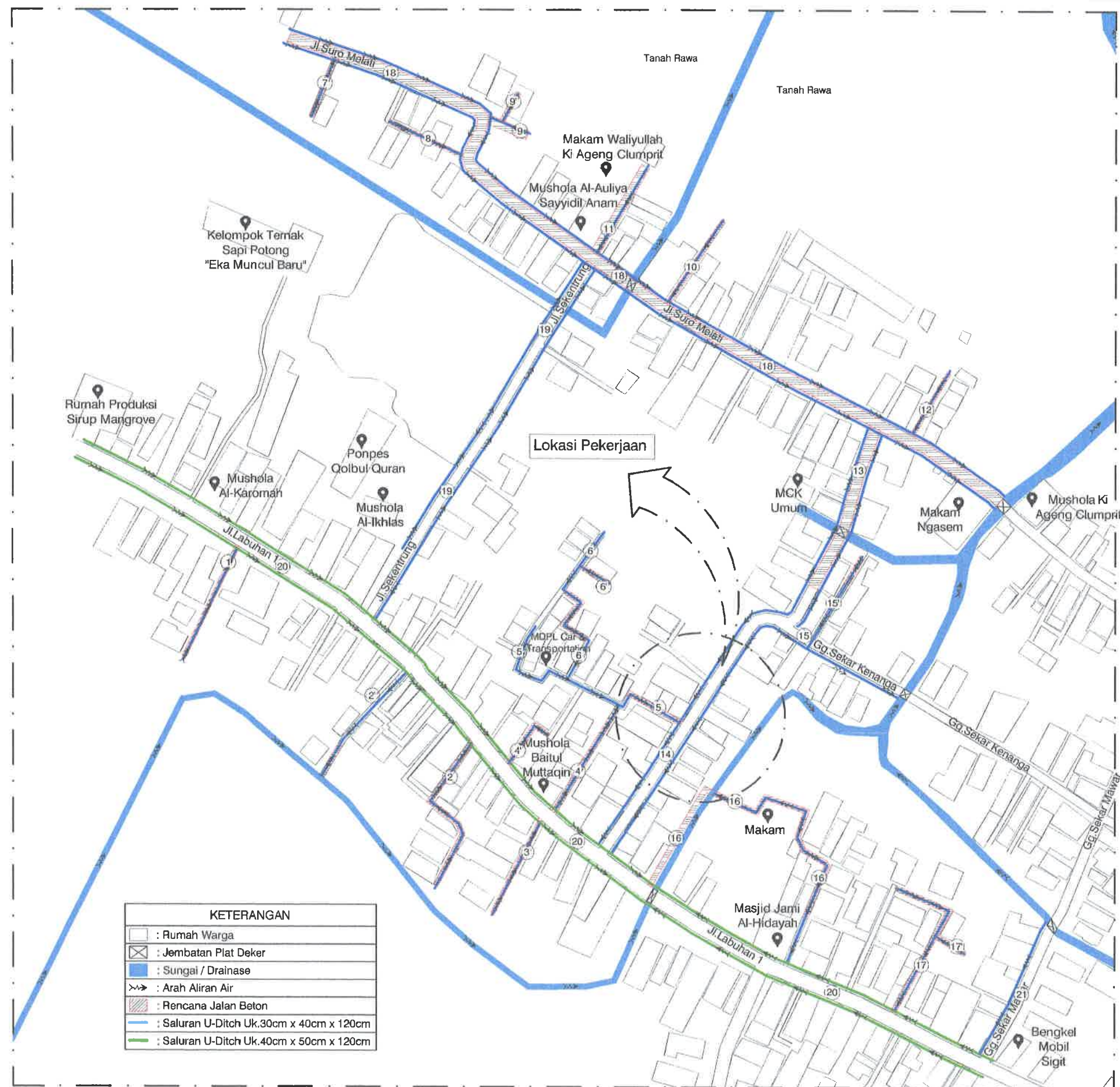
SITEPLAN RENCANA JALAN SALURAN DRAINASE RUAS 14 SKALA : Nis
