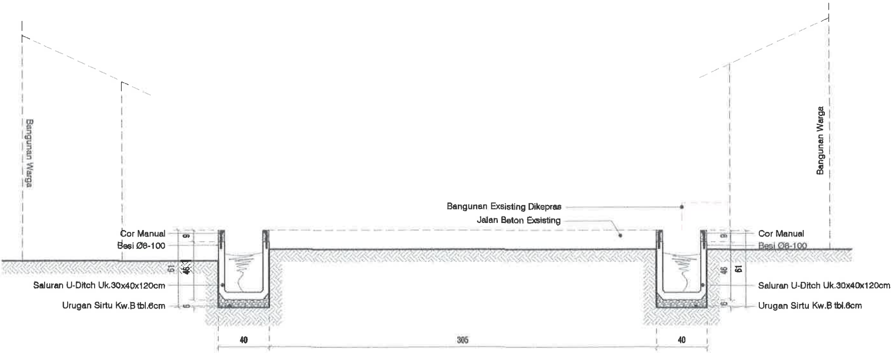
POTONGAN STA 0+100 SKALA 1 : 30
