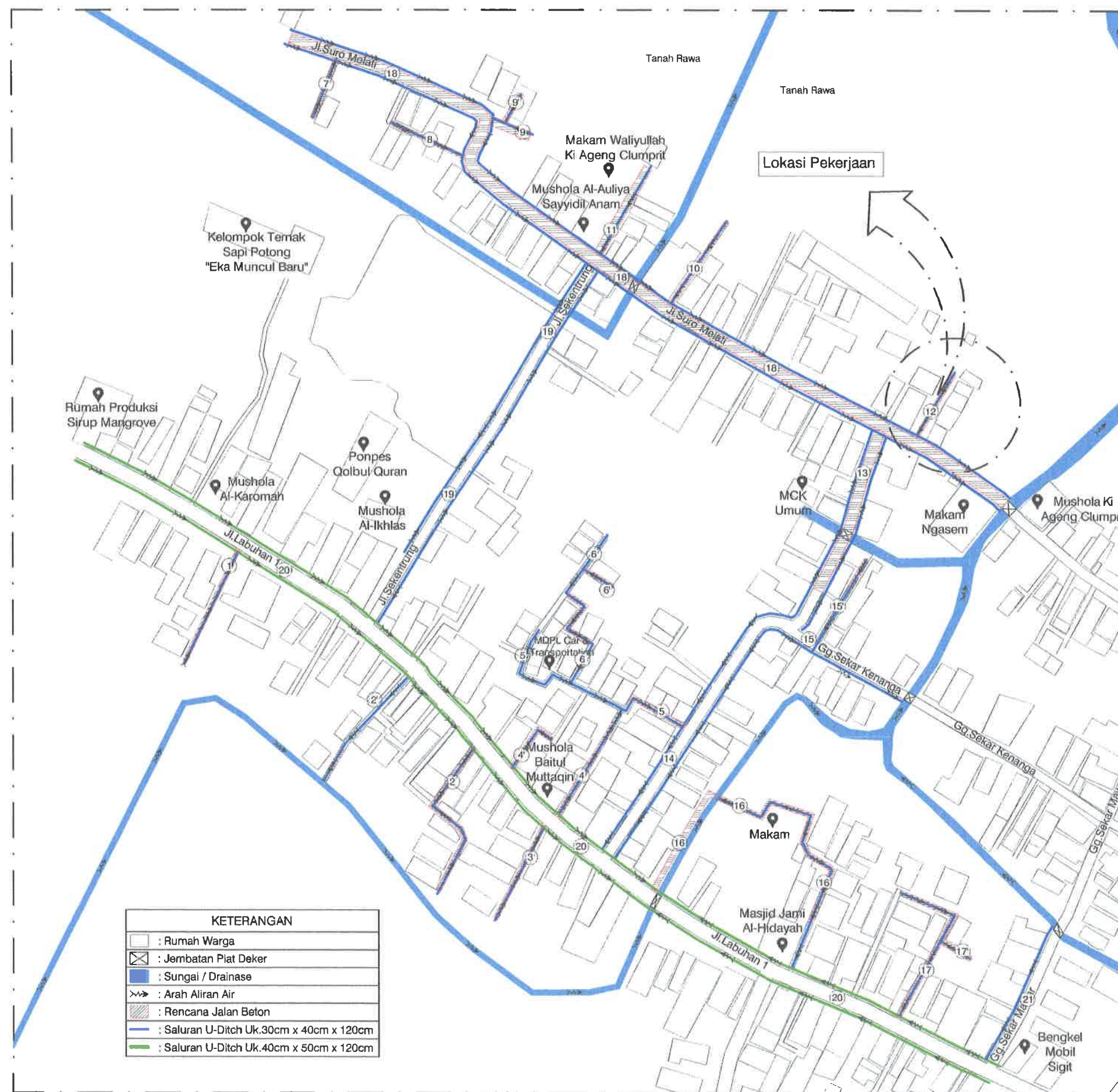
SITEPLAN RENCANA JALAN SALURAN DRAINASE RUAS 12 SKALA : Nis
