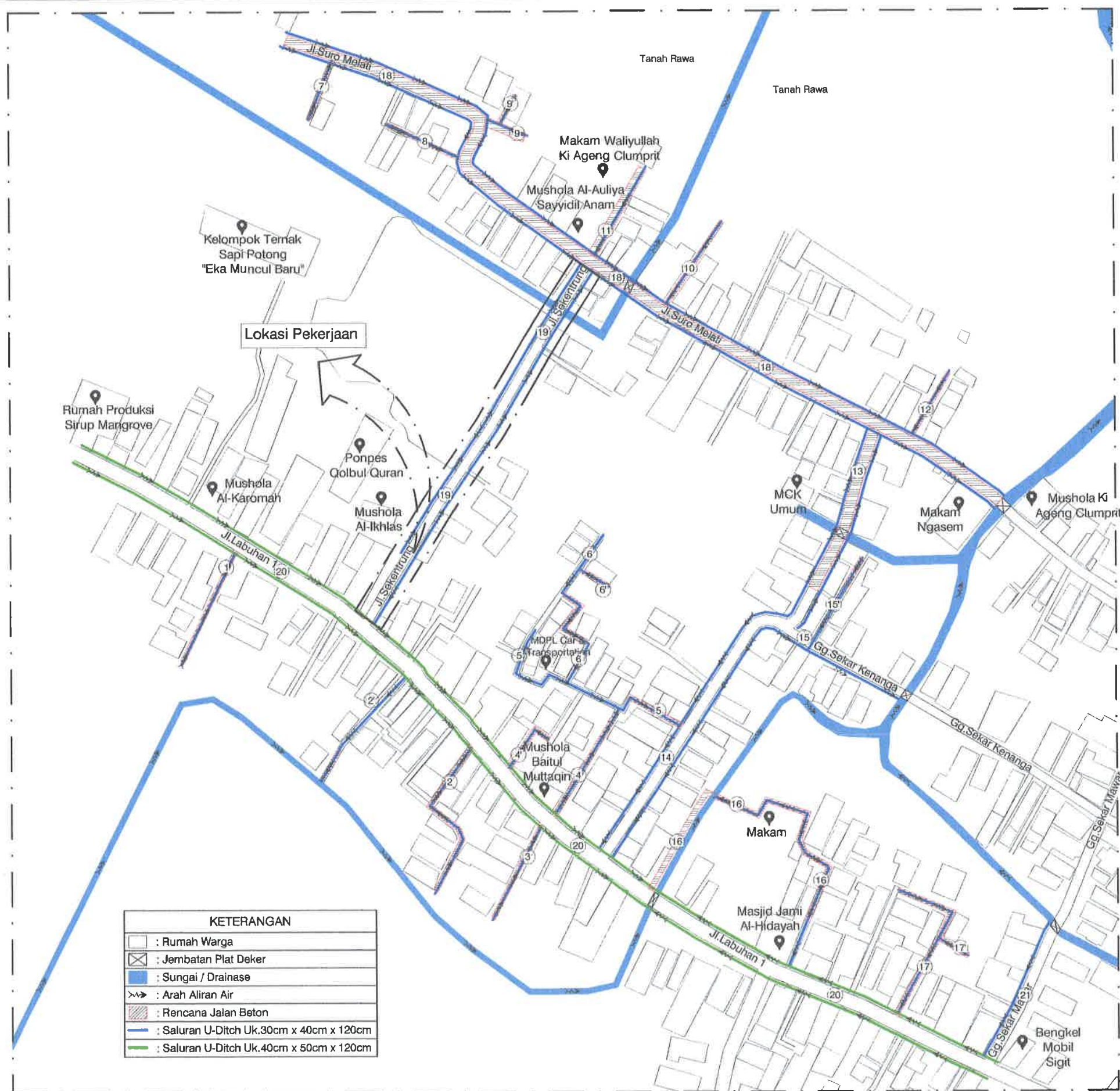
SITEPLAN RENCANA SALURAN DRAINASE RUAS 19
