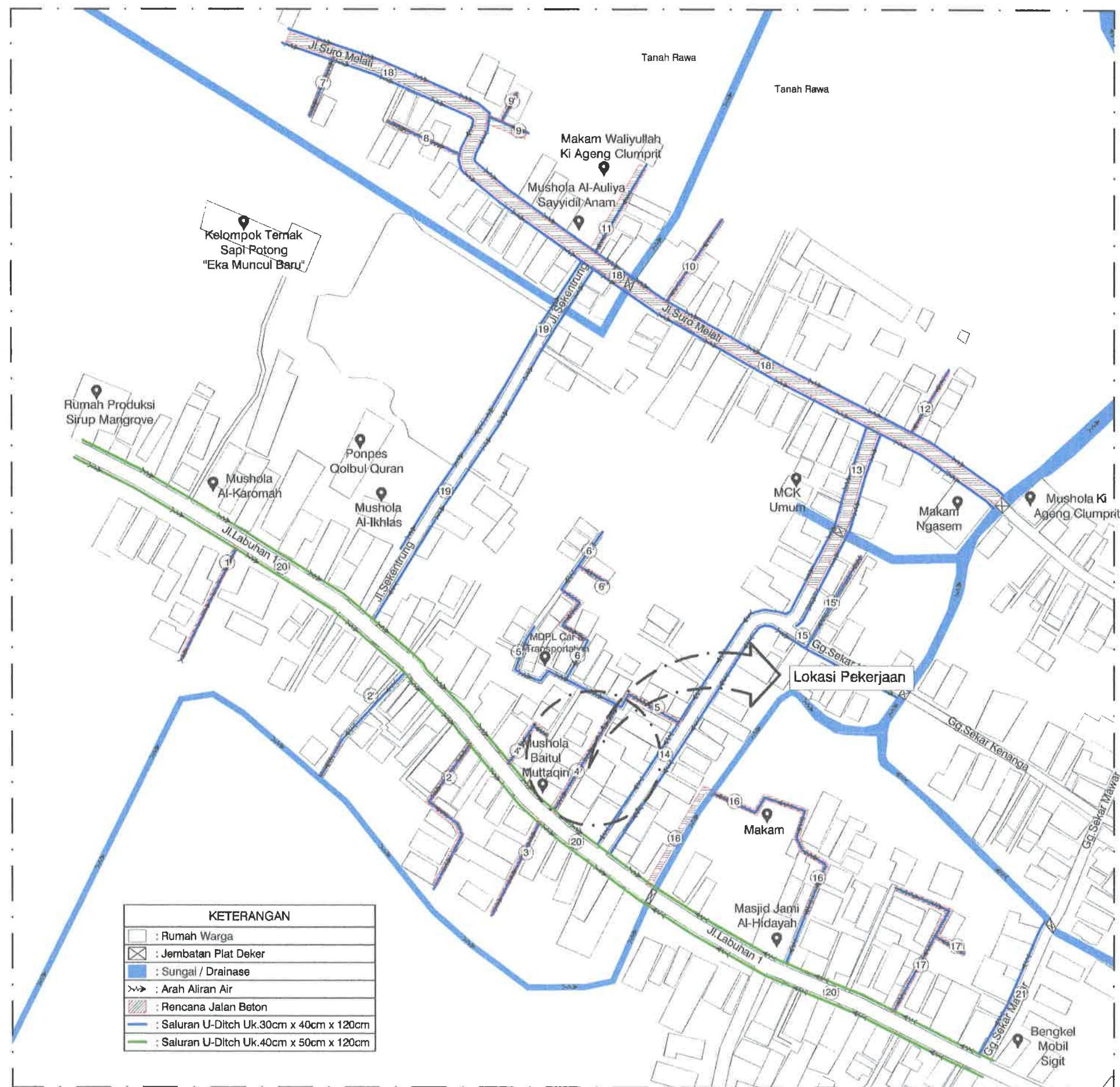
SITEPLAN RENCANA JALAN SALURAN DRAINASE RUAS 4 SKALA : Nts
