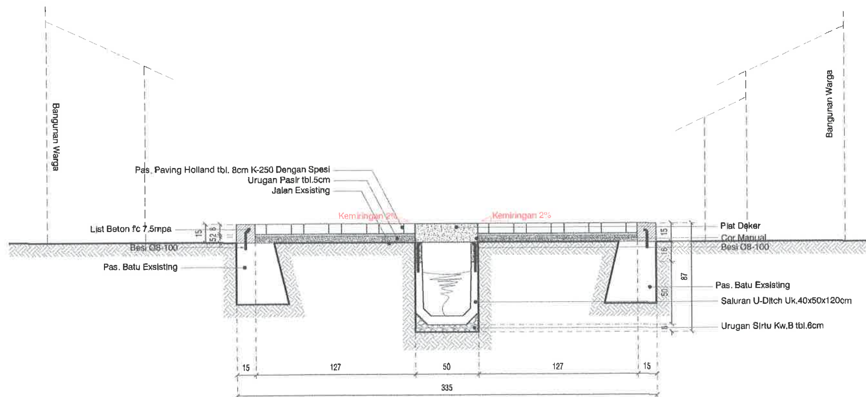
POTONGAN STA 0+175 SKALA 1 : 30
