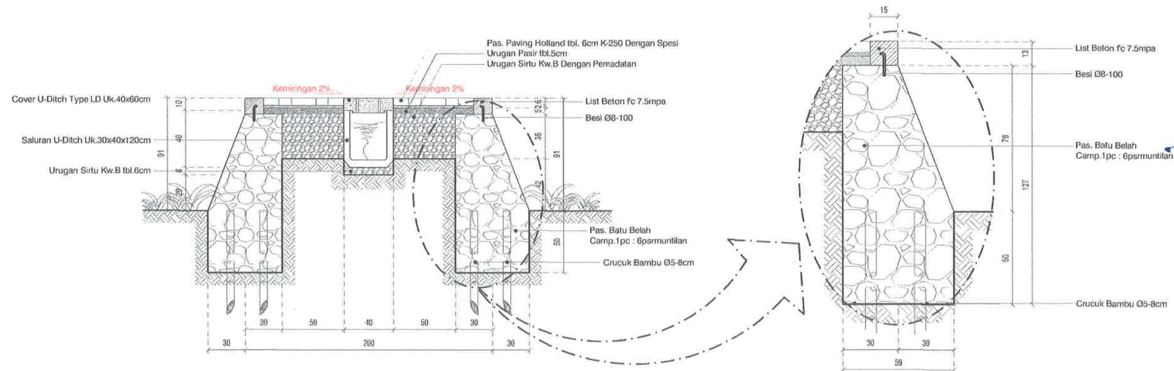
POTONGAN STA 0+016.5 SKALA 1 : 30
