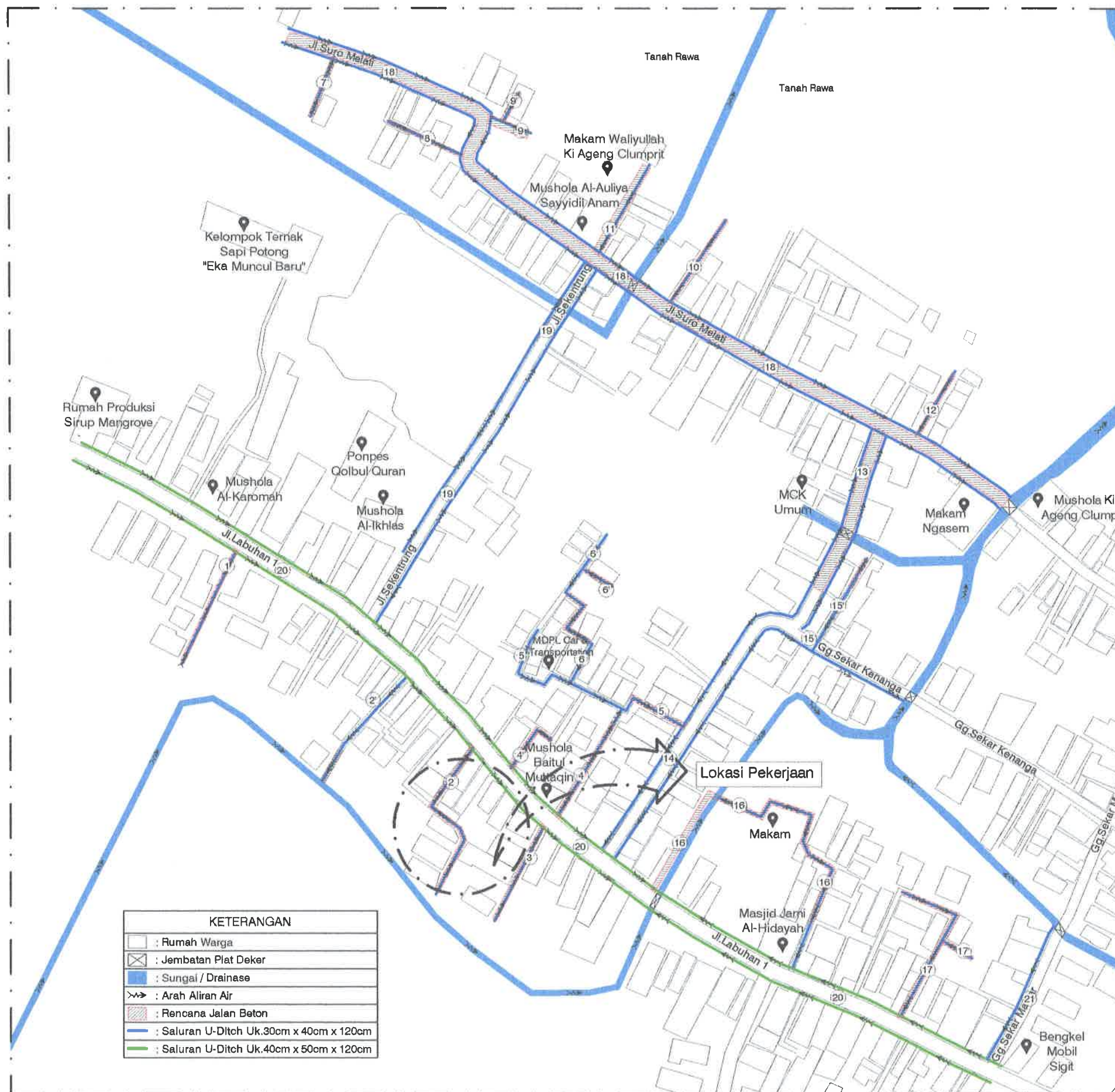
SITEPLAN RENCANA JALAN DAN SALURAN DRAINASE RUAS 2 SKALA : Nts
