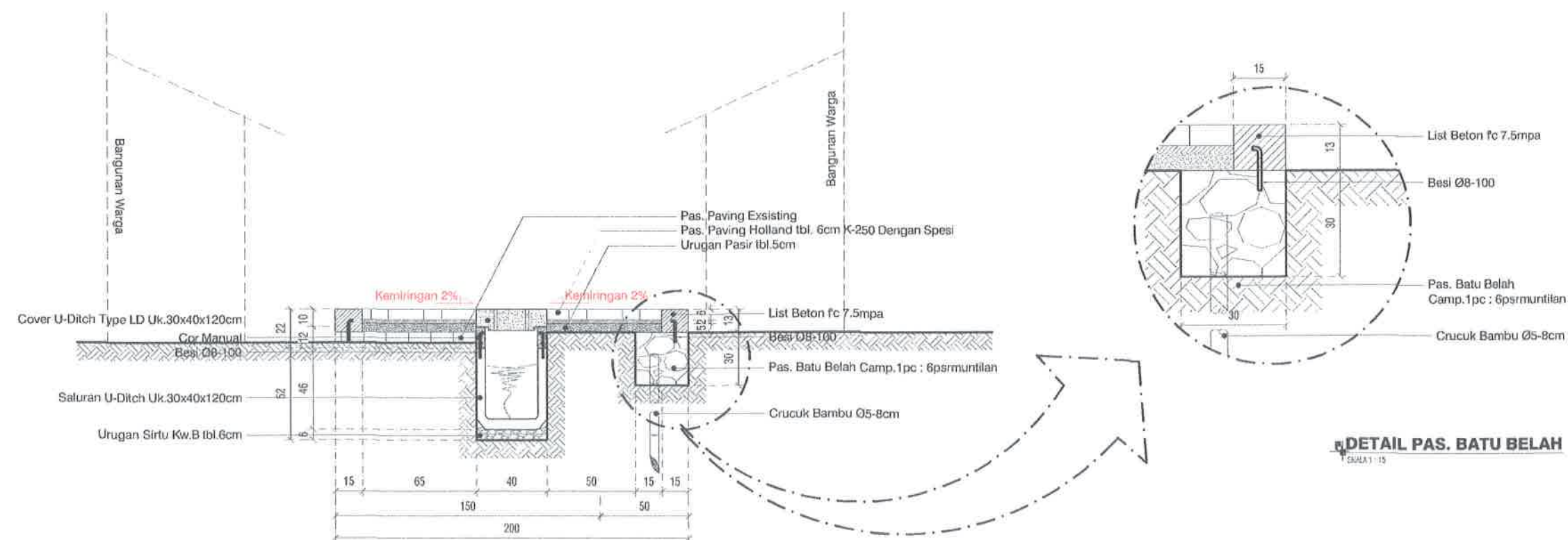
POTONGAN STA 0+042.6
