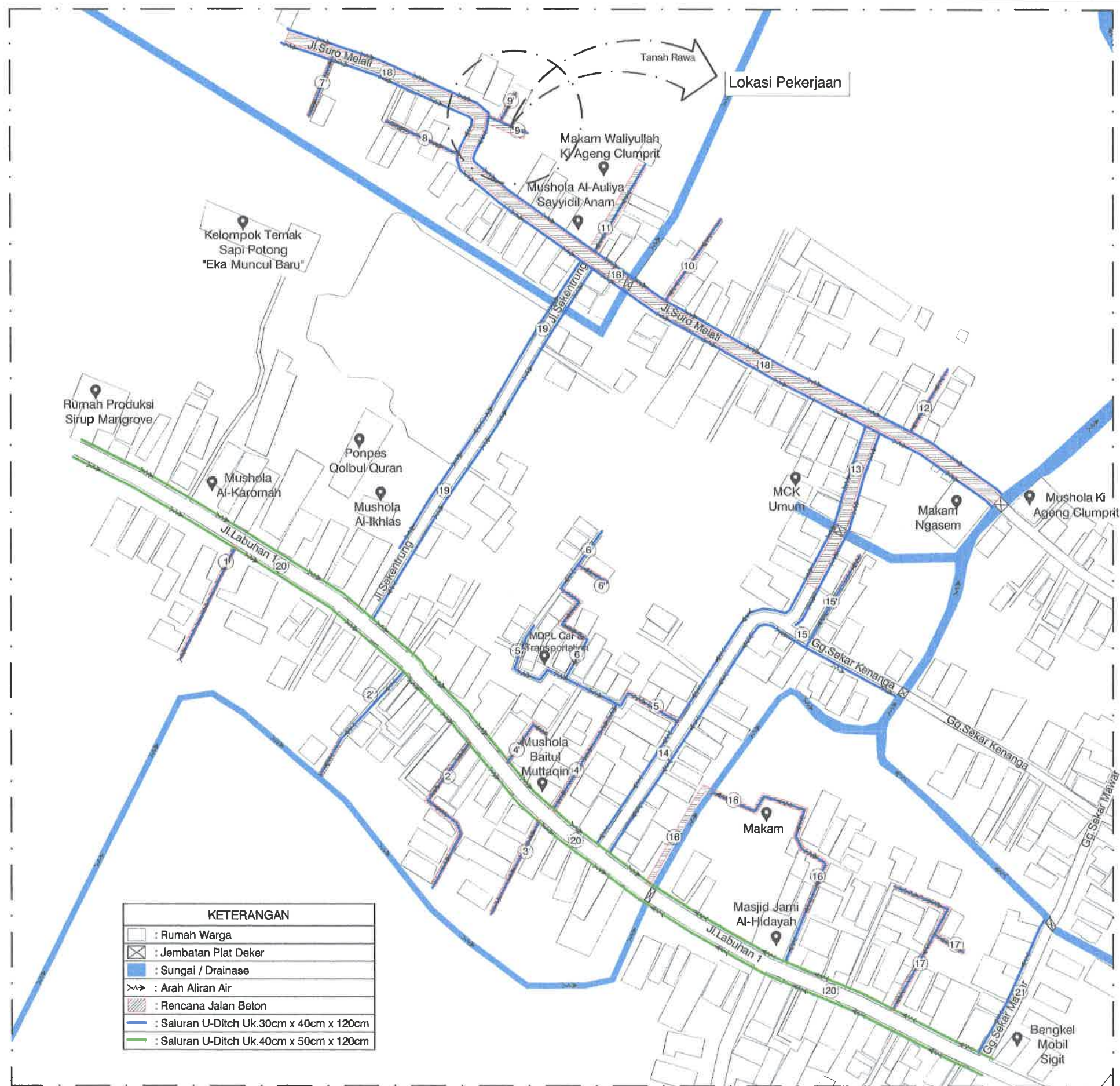
SITEPLAN RENCANA JALAN SALURAN DRAINASE RUAS 9 SKALA : Nis
