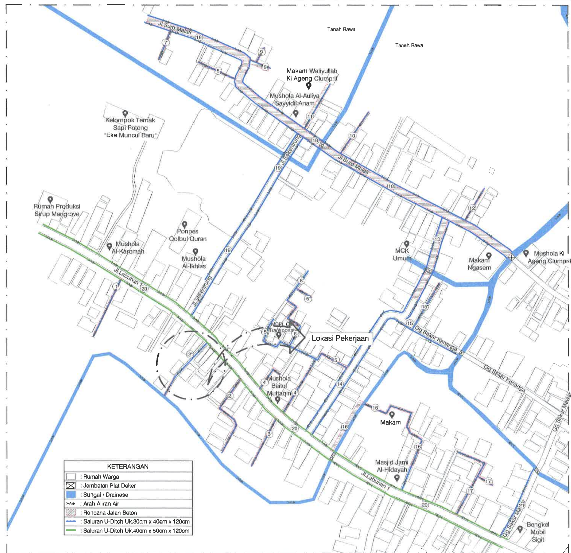
SITEPLAN RENCANA SALURAN DRAINASE RUAS 2' SKALA : NIS
