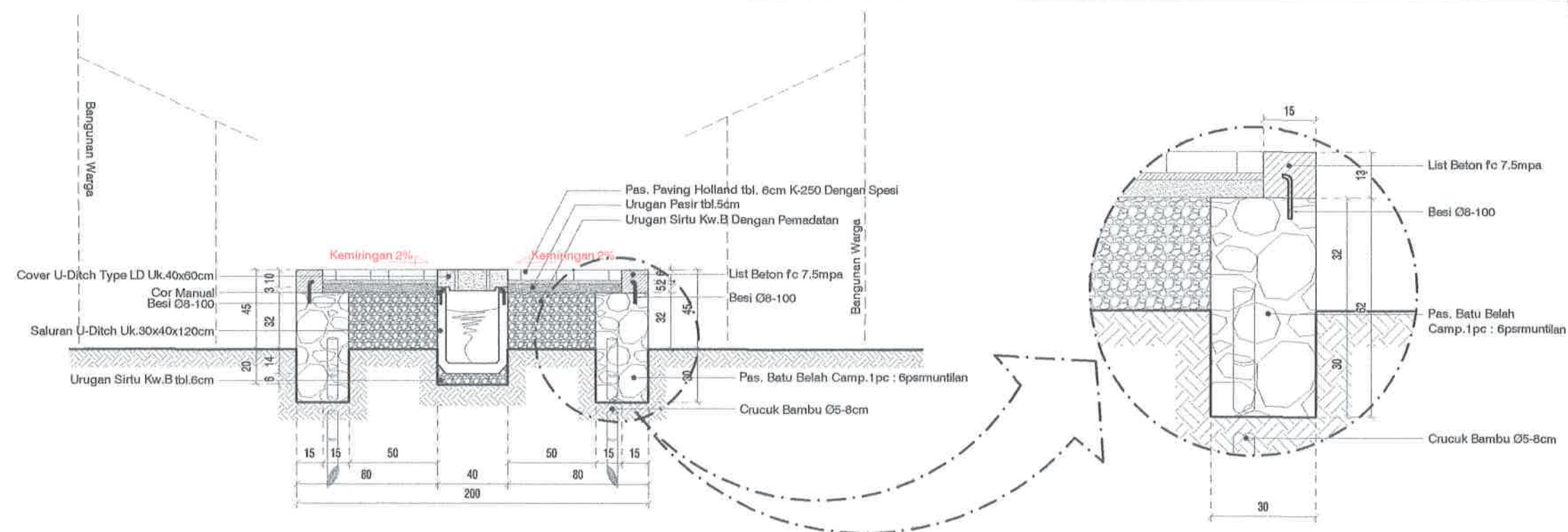
DETAIL PAS. BATU BELAH SKALA 1 : 15
