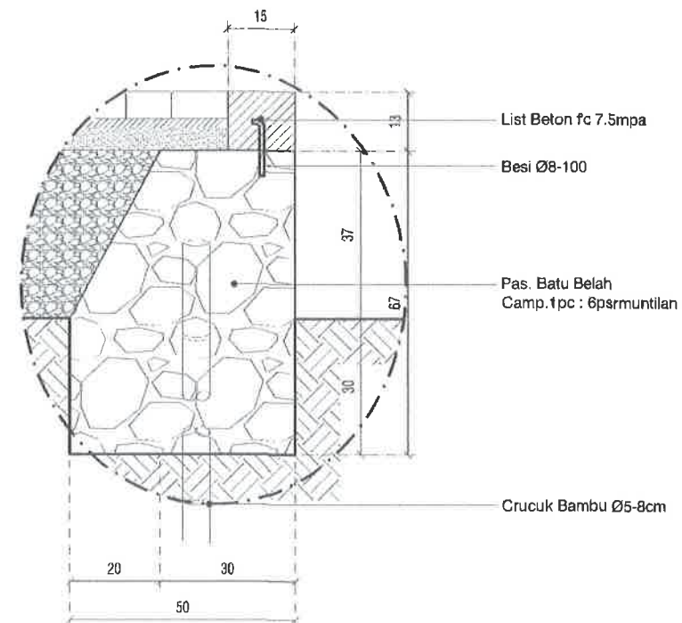
POTONGAN STA 0+025
