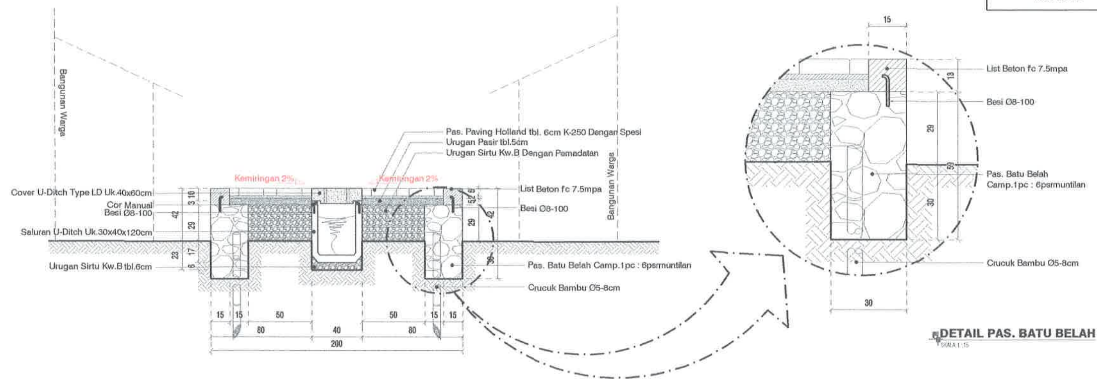
POTONGAN STA 0+032 SKALA 1 : 30
