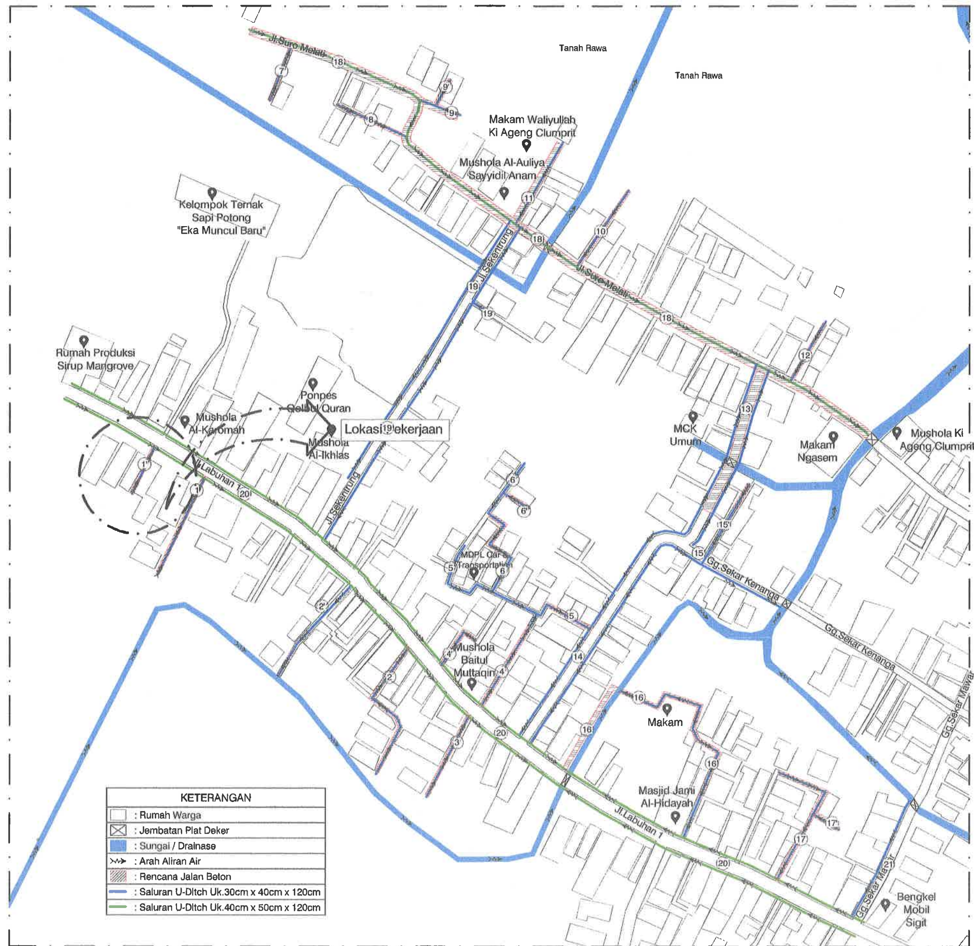
SITEPLAN RENCANA JALAN DAN SALURAN DRAINASE RUAS 1' SKALA : Nts
