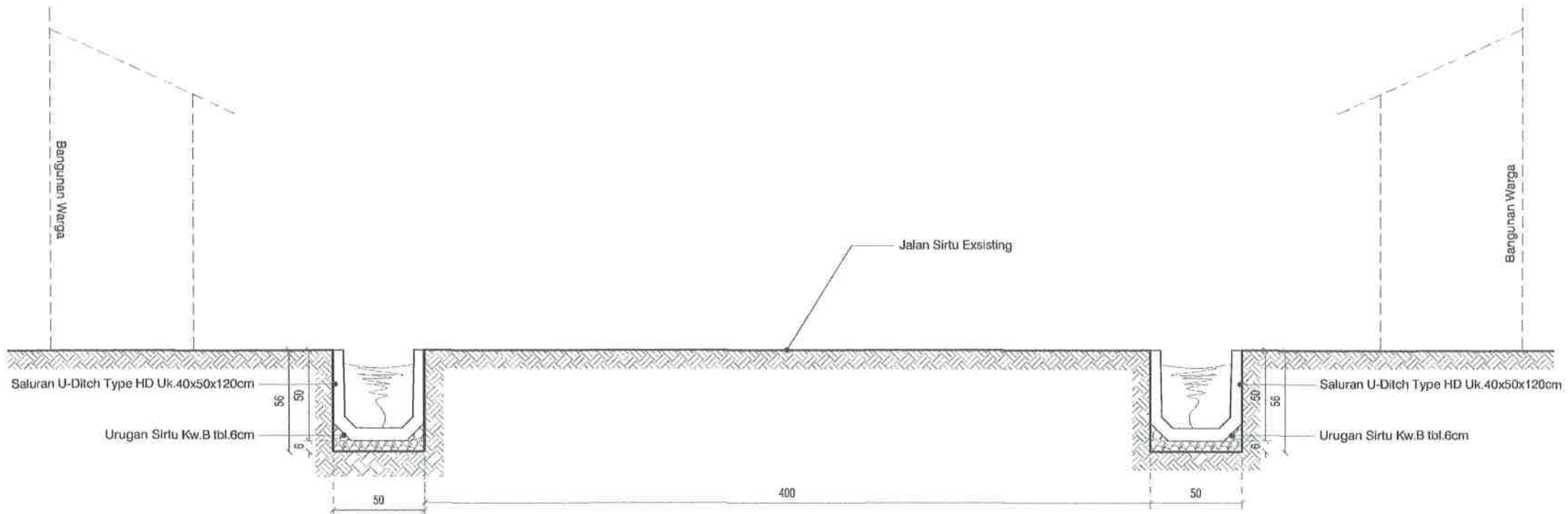
POTONGAN STA 0+450 SKALA 1 : 30
