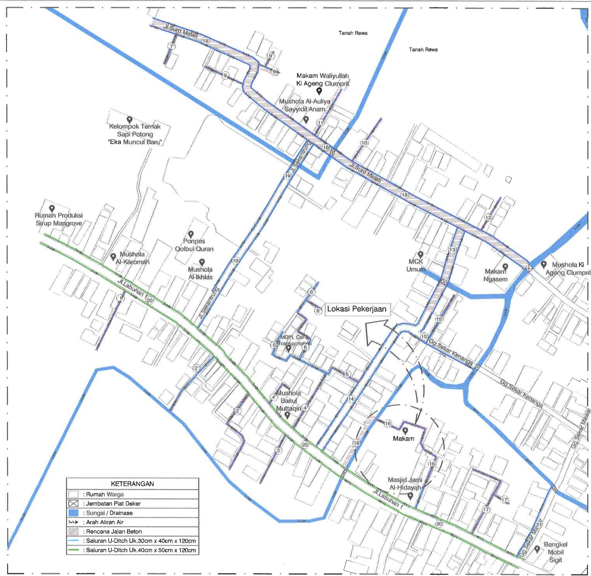
SITEPLAN RENCANA JALAN SALURAN DRAINASE RUAS 16 SKALA : Nis
