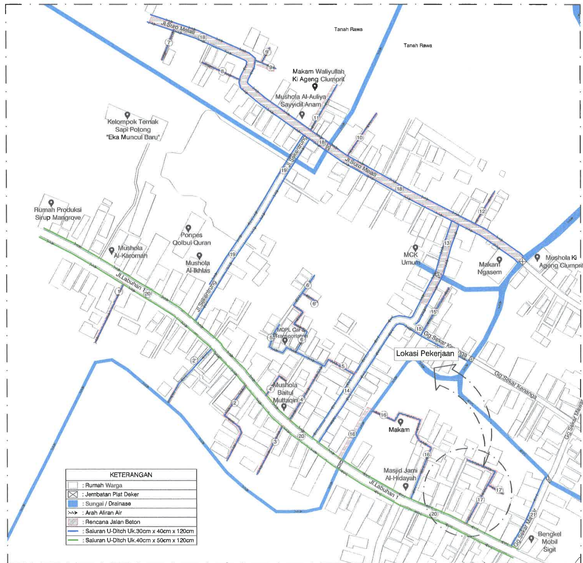
SITEPLAN RENCANA JALAN SALURAN DRAINASE RUAS 17
