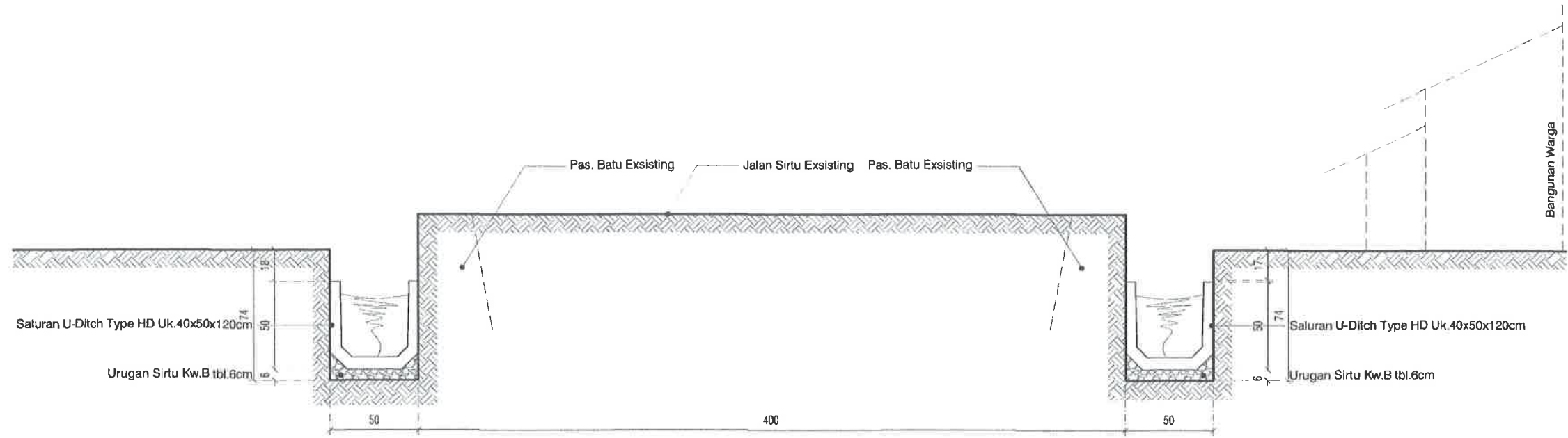
POTONGAN STA 0+000
