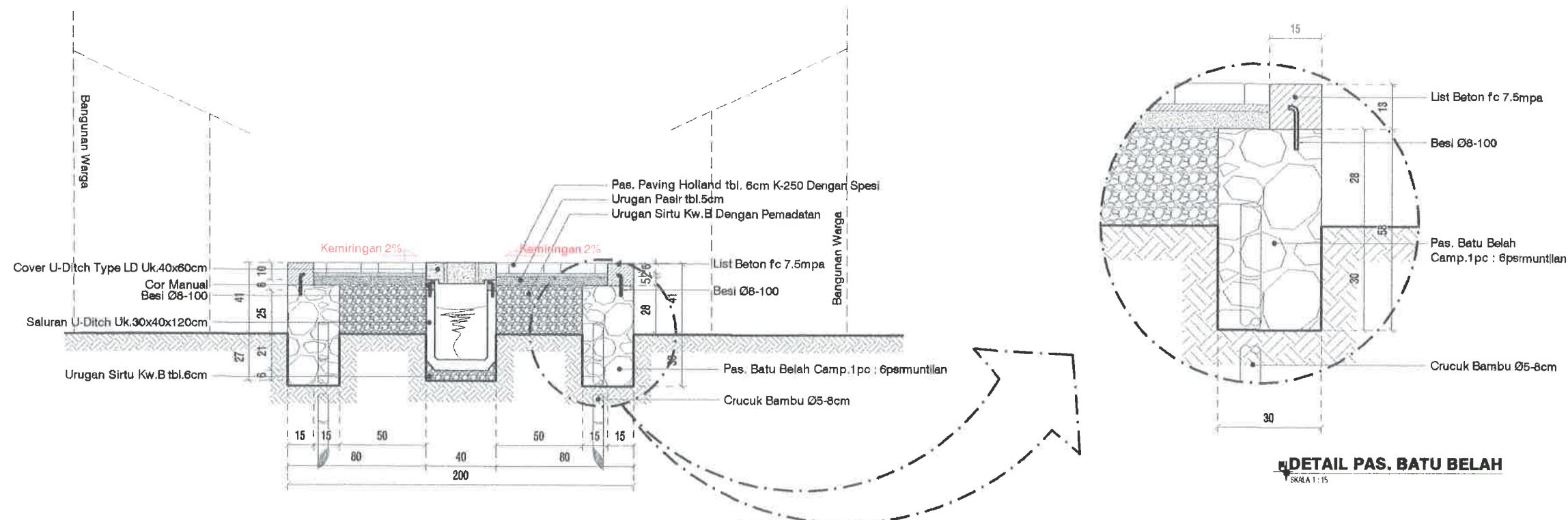
POTONGAN STA 0+027 SKALA 1 : 30
