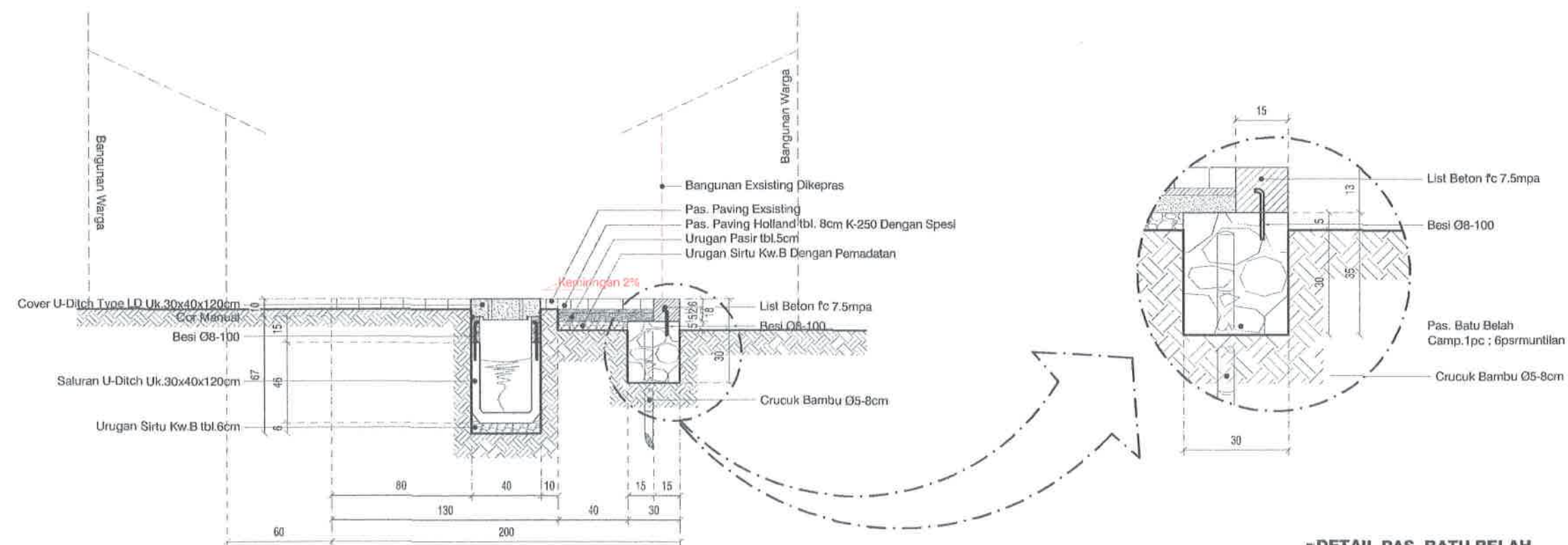
POTONGAN STA 0+028.2
