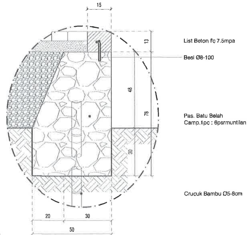
POTONGAN STA 0+015.4 SKALA 1 : 30
