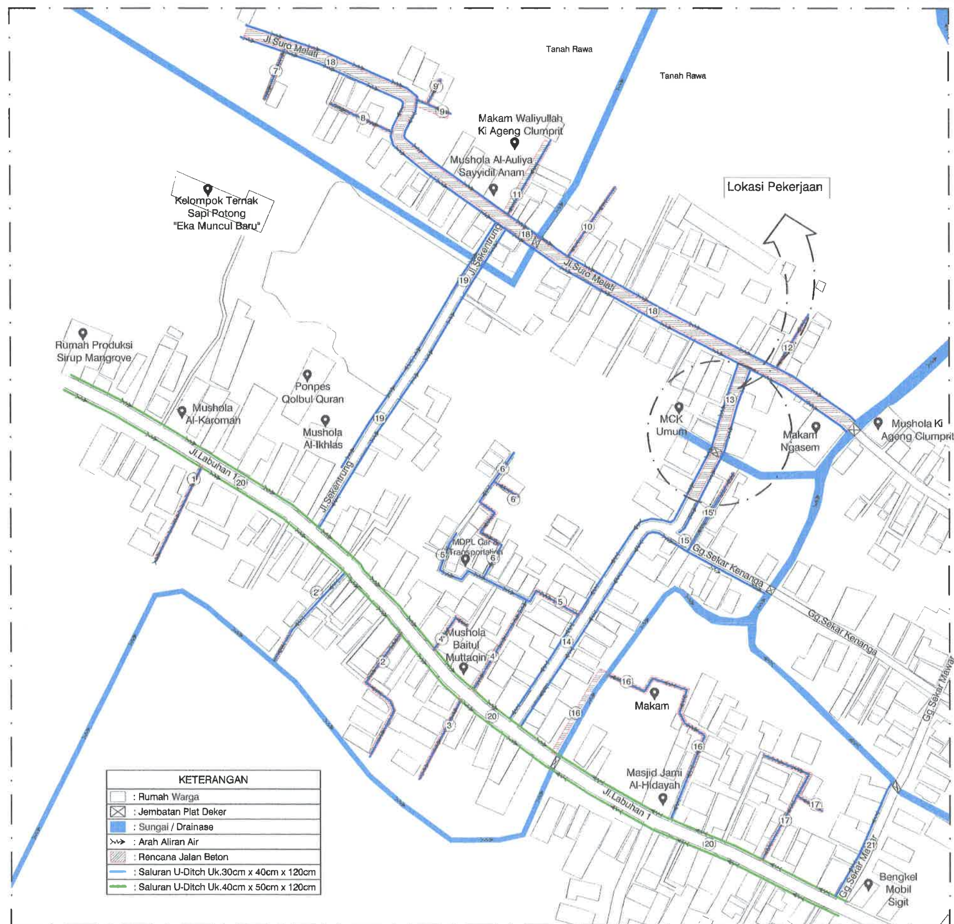
SITEPLAN RENCANA JALAN SALURAN DRAINASE RUAS 13 SKALA : Nis
