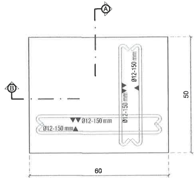
PLAT DEKER TAMPAK ATAS
